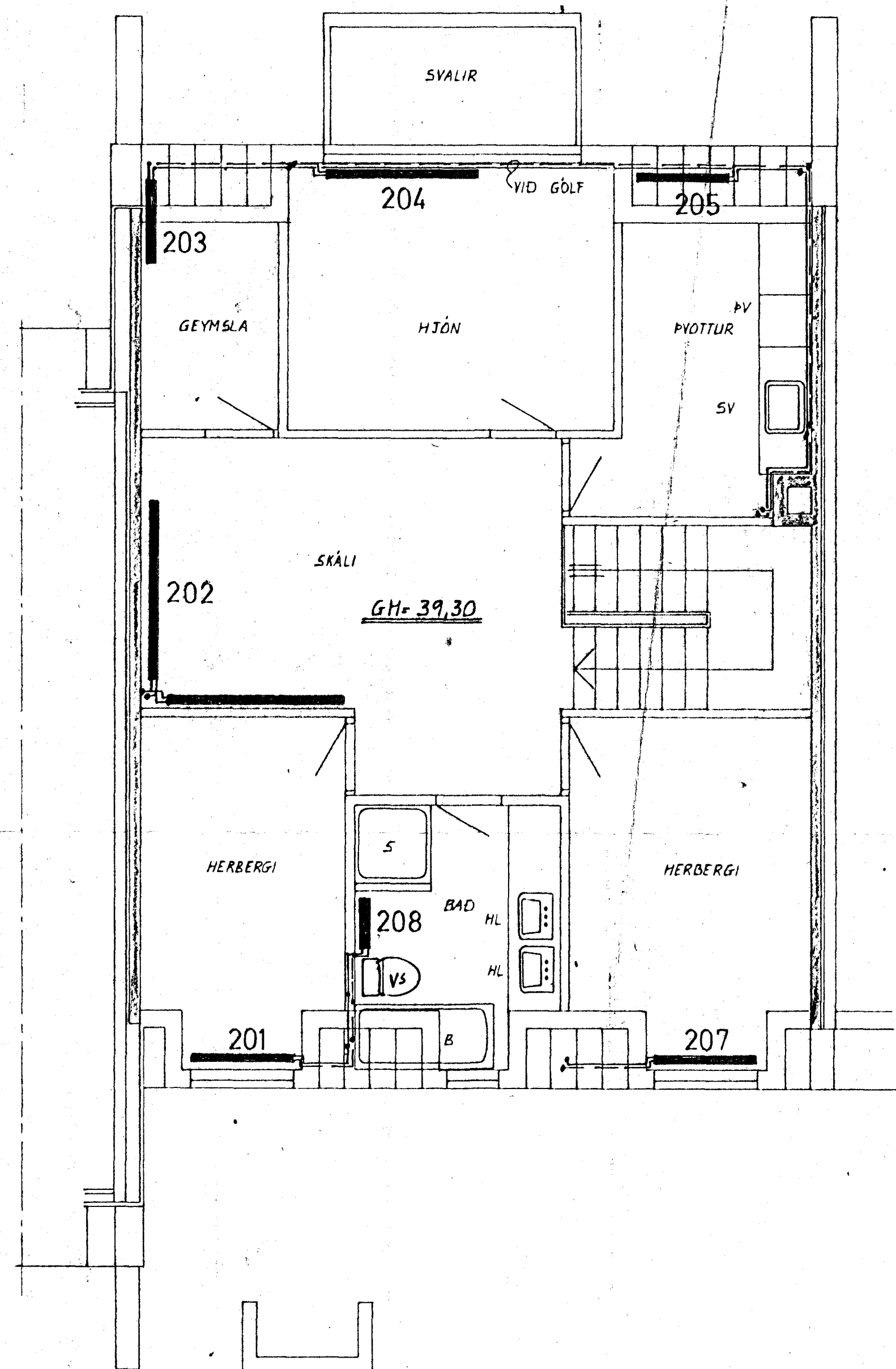
GRUNNMYND - 1. HÆÐ 1:50
