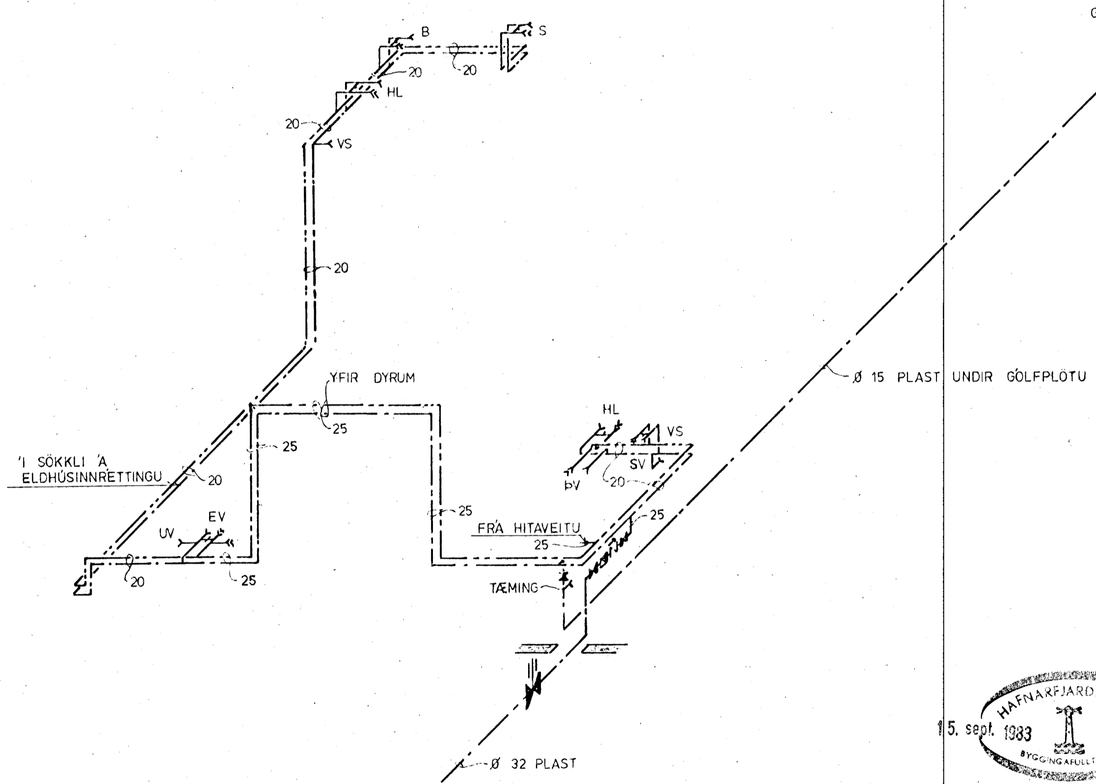
KERFI ~ 1 : 50
