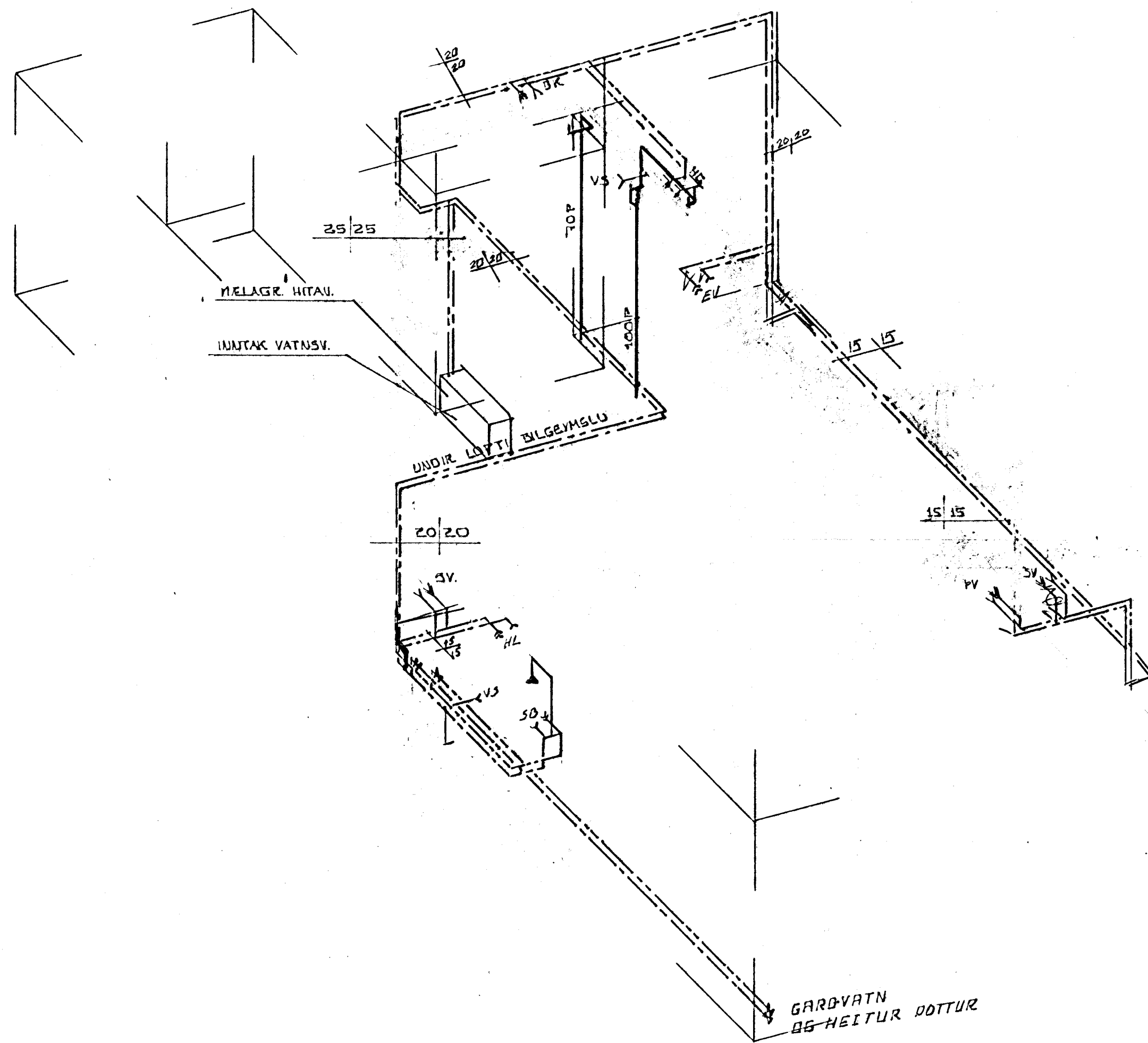
RÚMMYND 1:50
