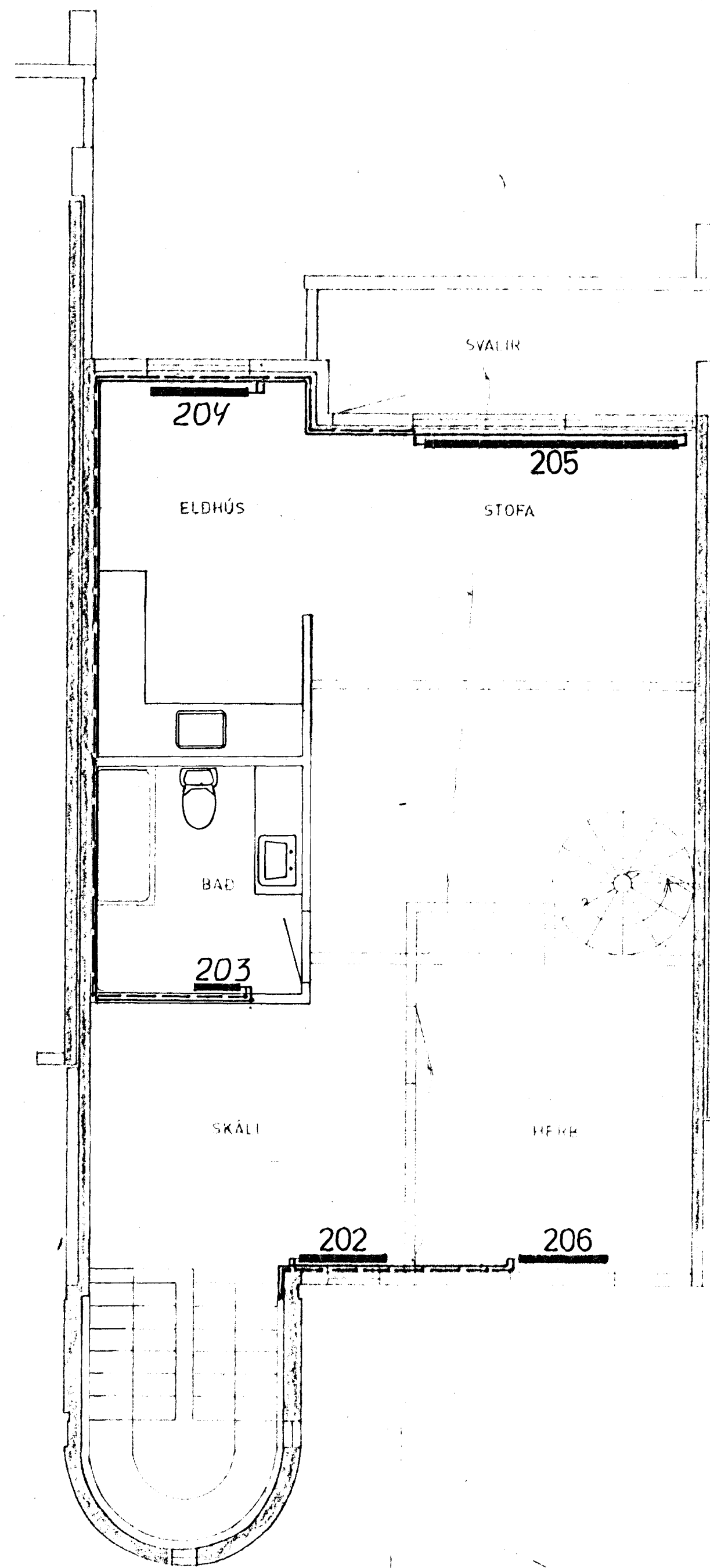
GRUNNMYND 2. HÆÐAR 1:50
