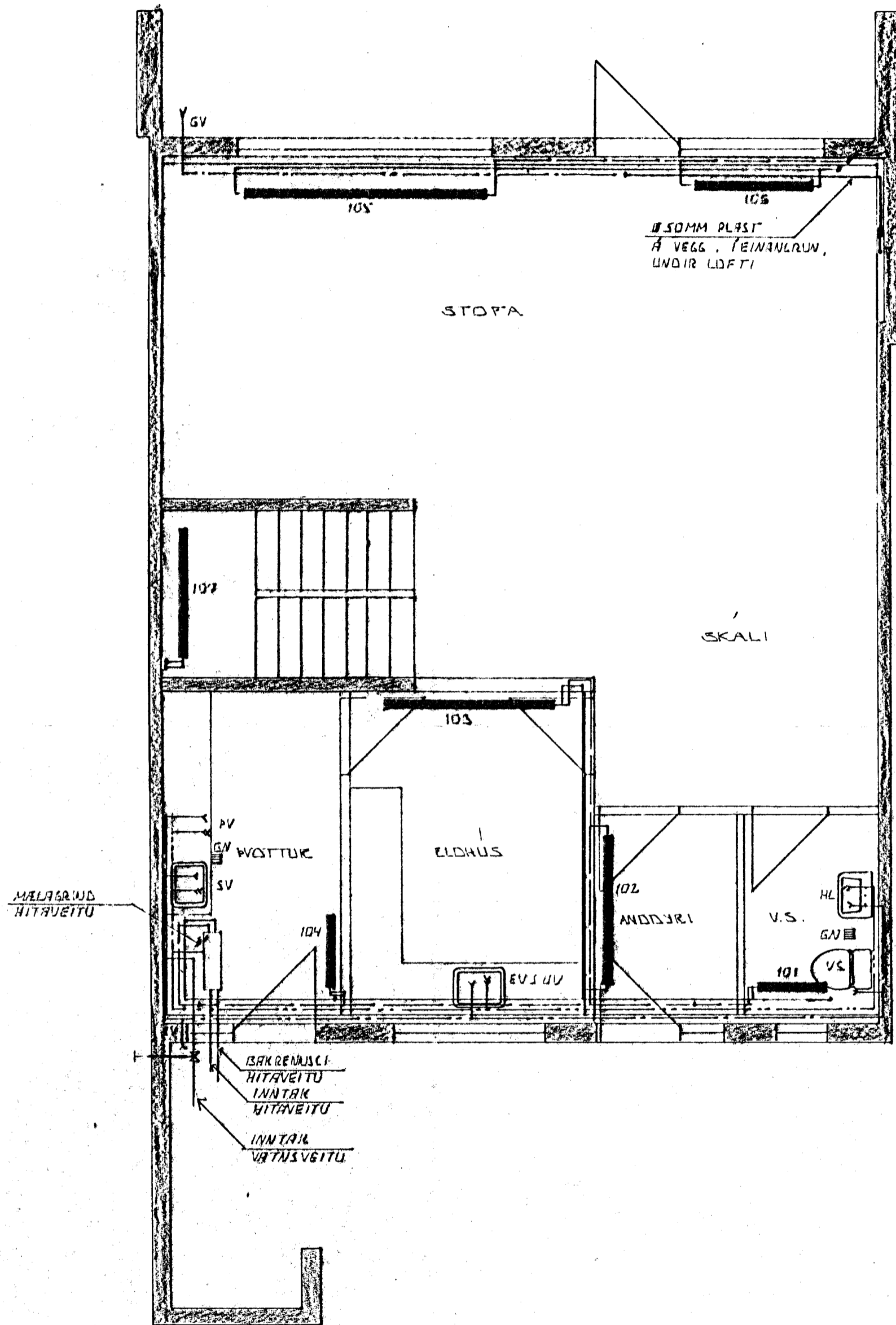
GRUNNMYND ~ 1:50
