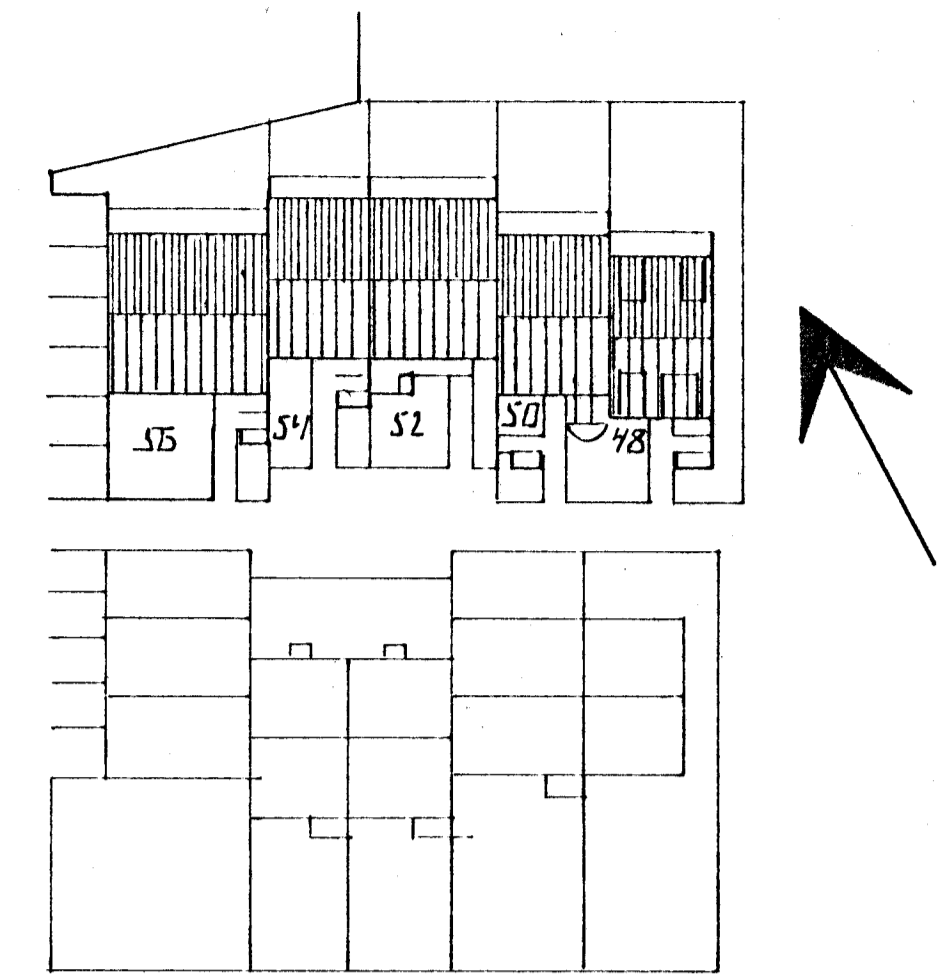
AFSTÖÐUMYND 1:500
