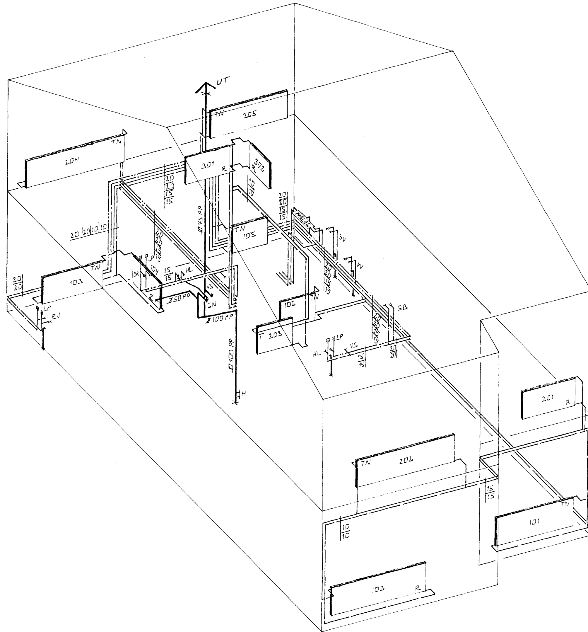
RÚMMYND 1:50
