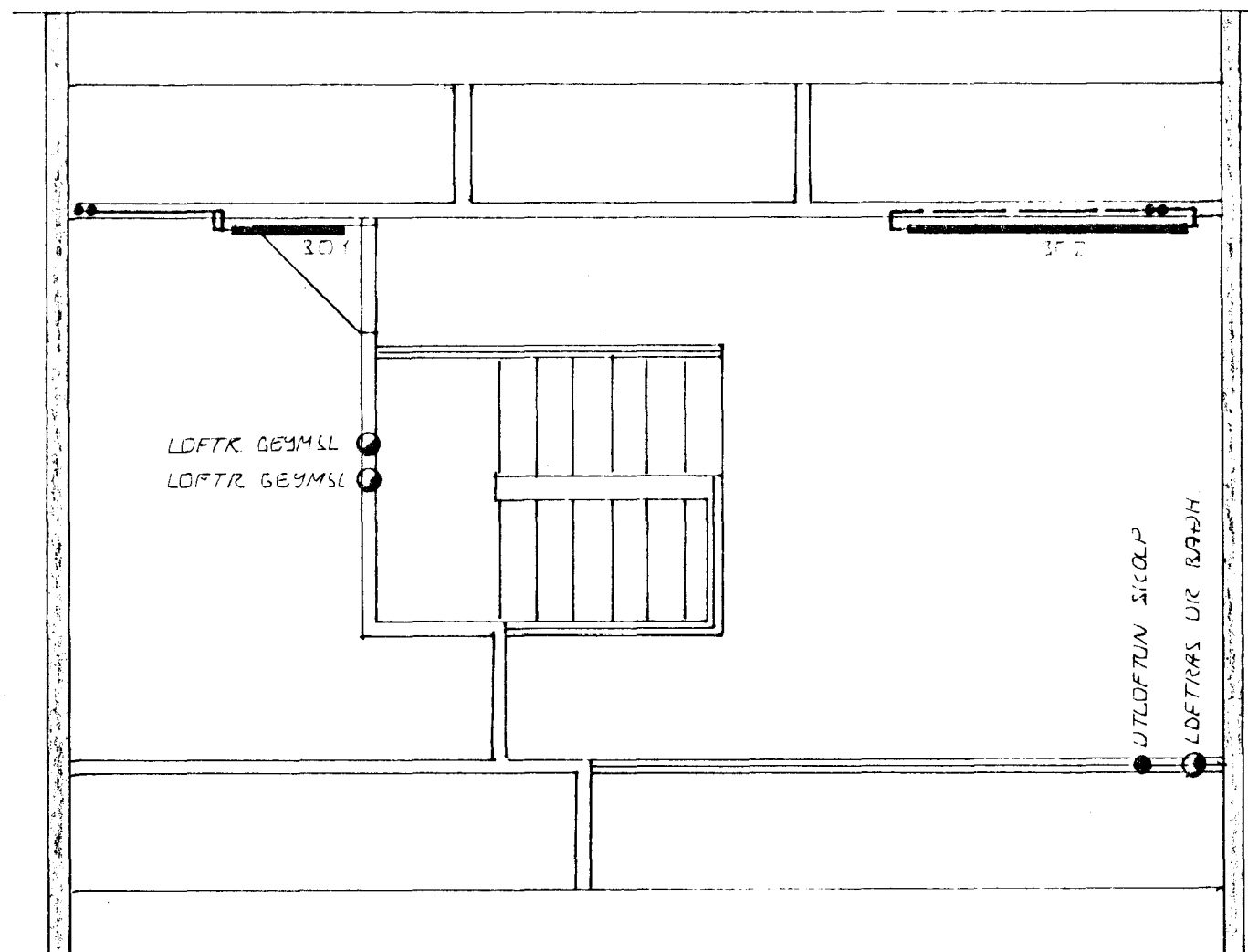
GRUNNMYND R1S ~1:50
