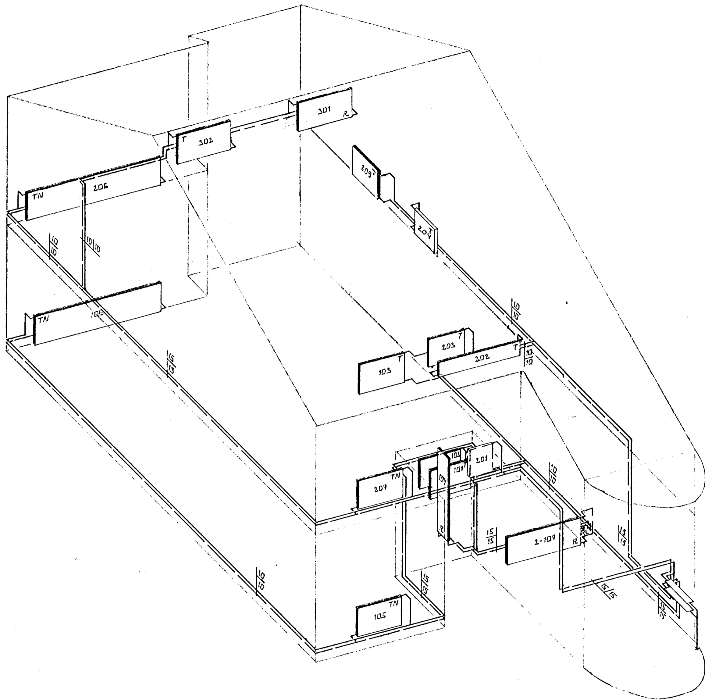
RÚMMYND 1:50
