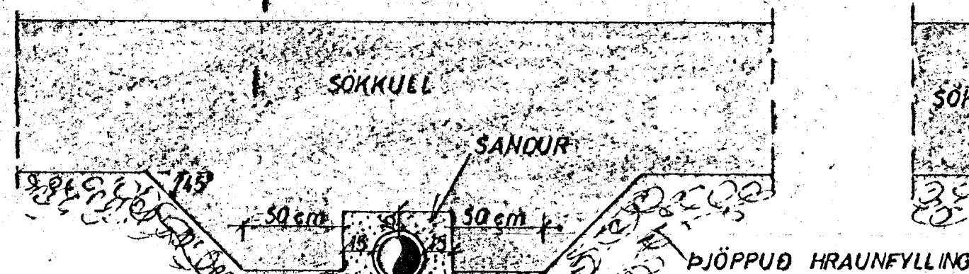
GRAFID SKAL FYRIR LÖGNUM UNDIR SÖKKLUM, ADUR EN ÞEIR ERU STEYPTIR
