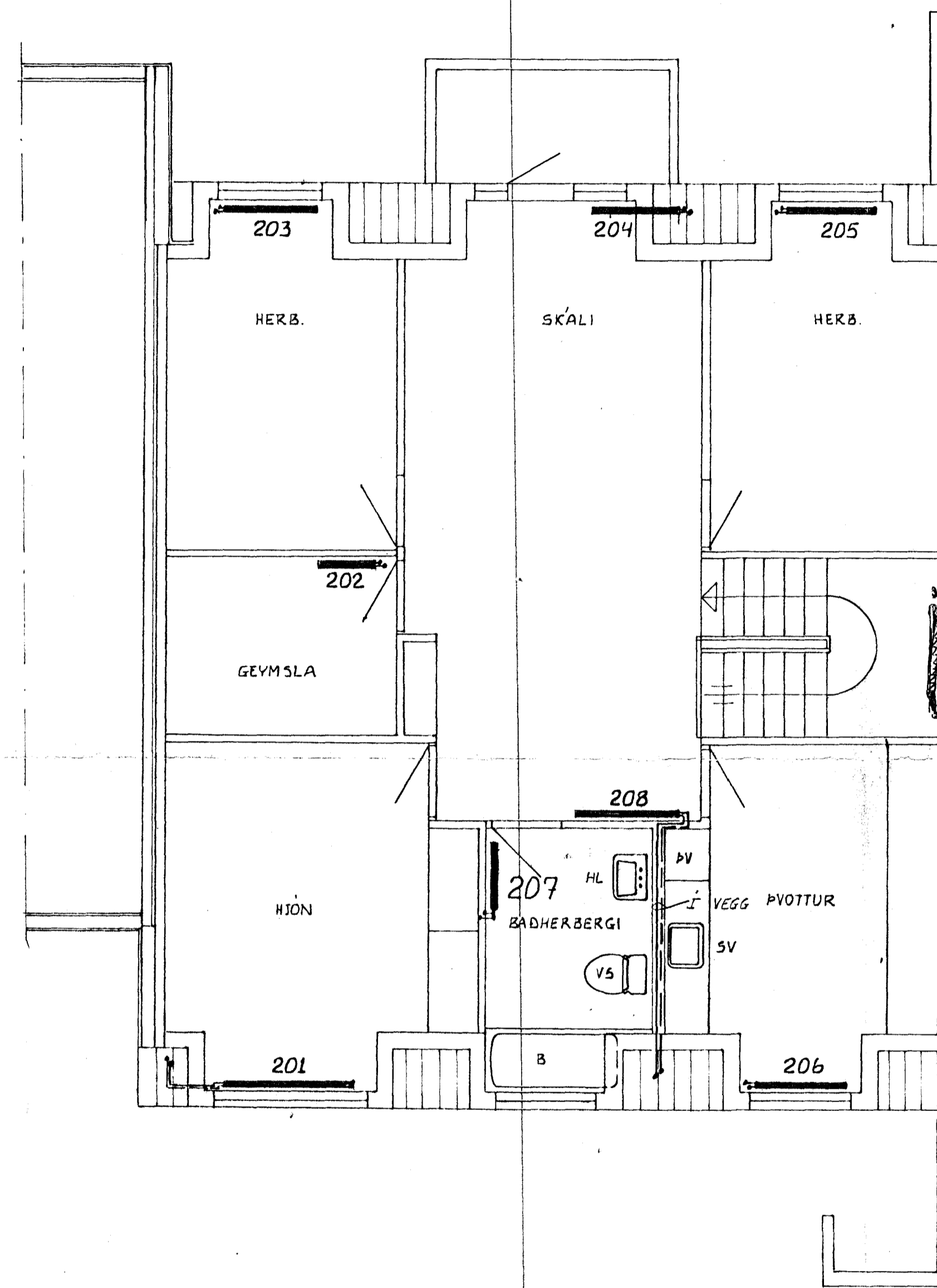
GRUNNMYND HÆÐAR 1:50
