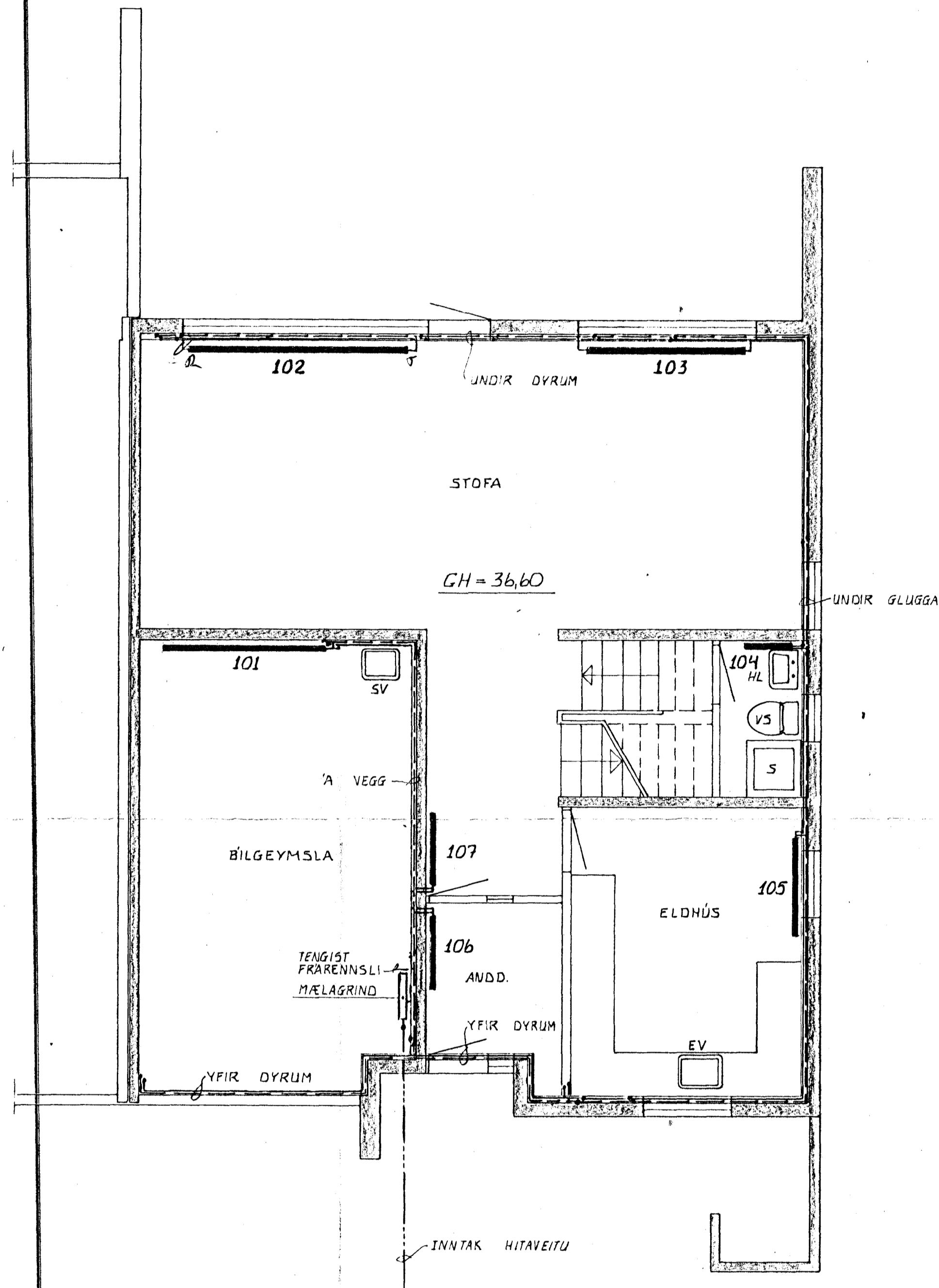
GRUNNMYND JARÐHÆÐ 1:50
