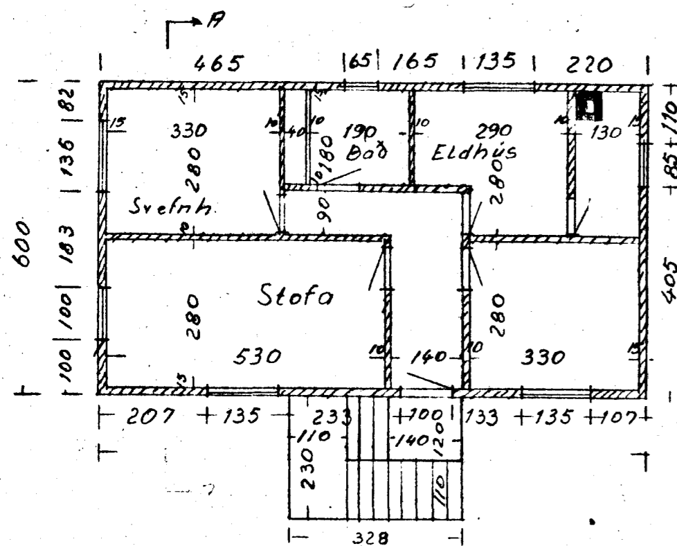
A Höð
