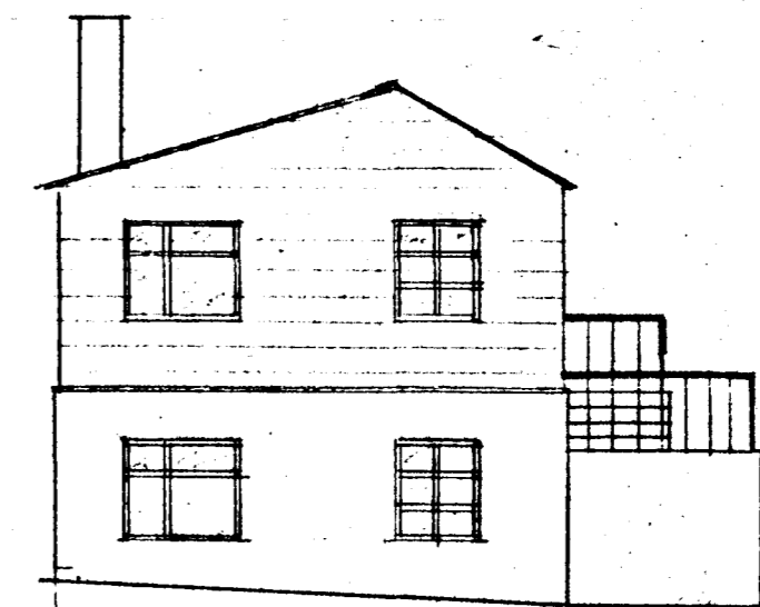
Suðaustur
