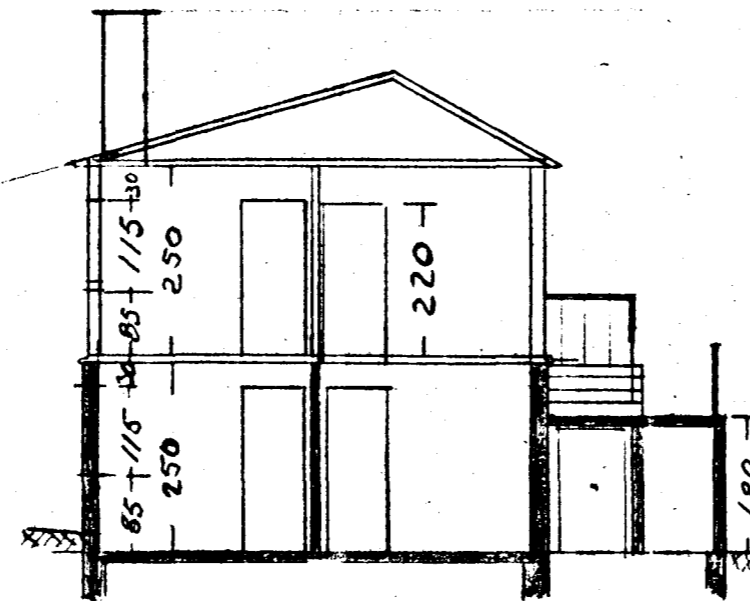
Snid A-A
