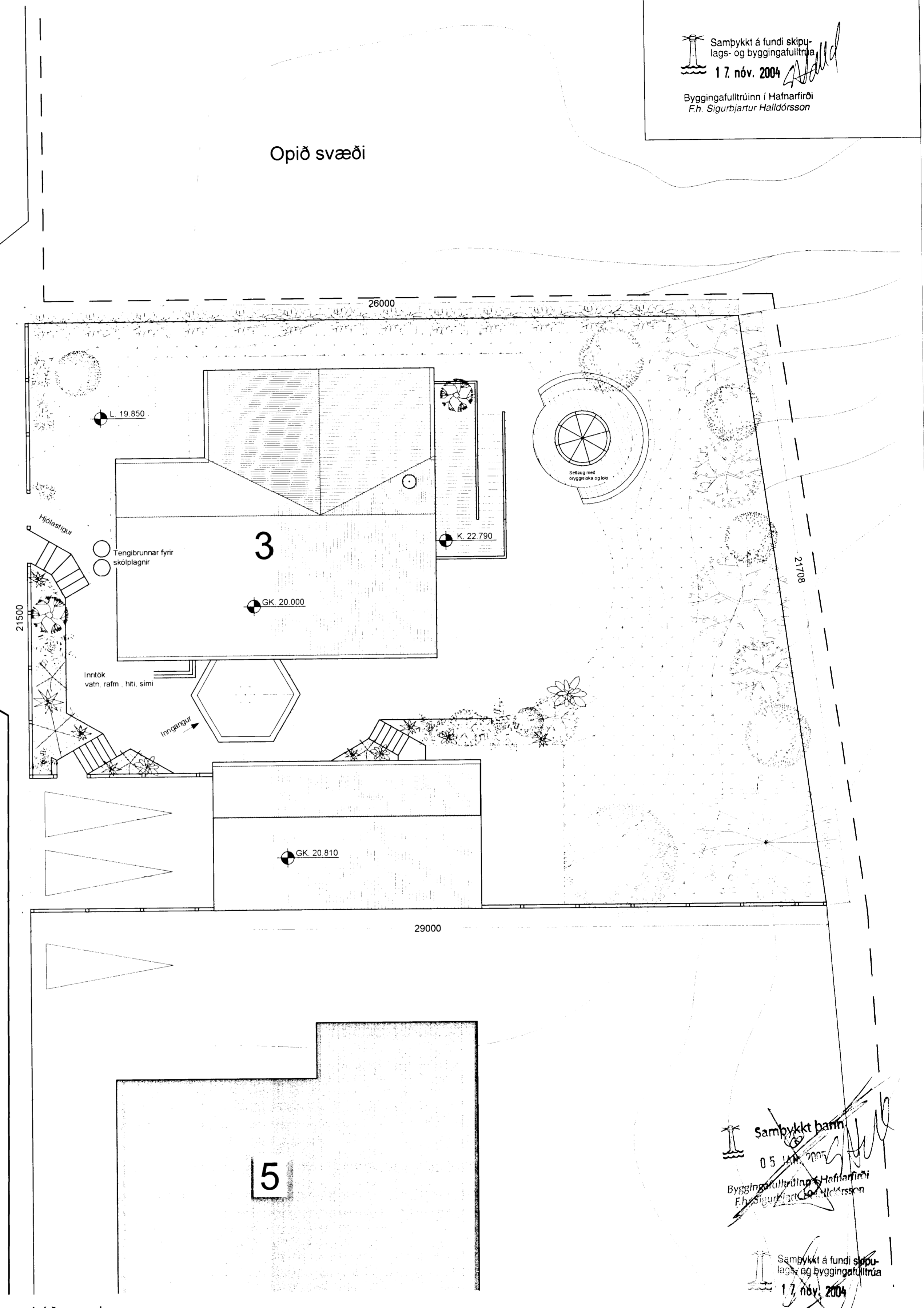
Lóðamynd Mál 1:100
