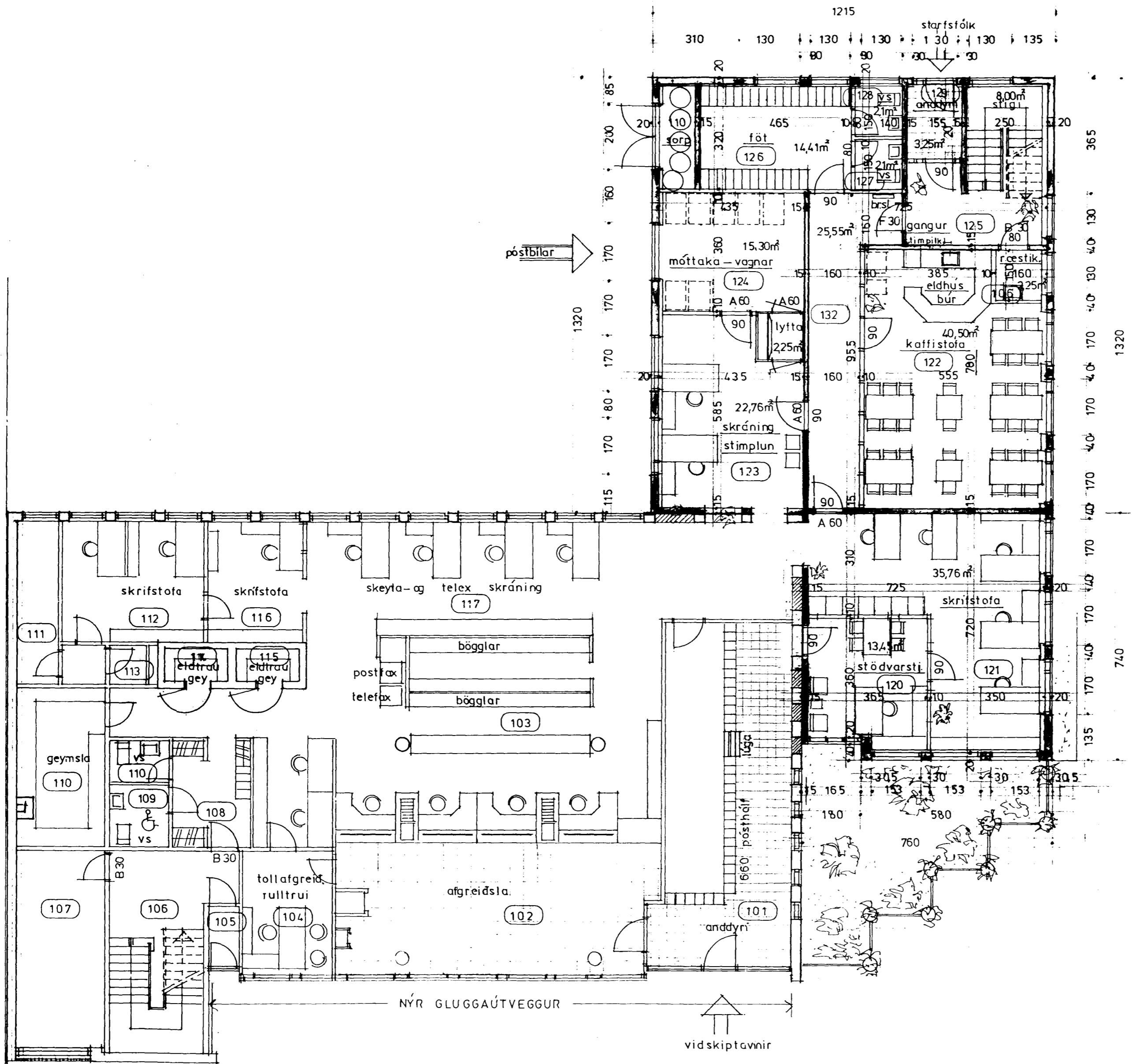
grunnmynd 1. hæðar 1:100
