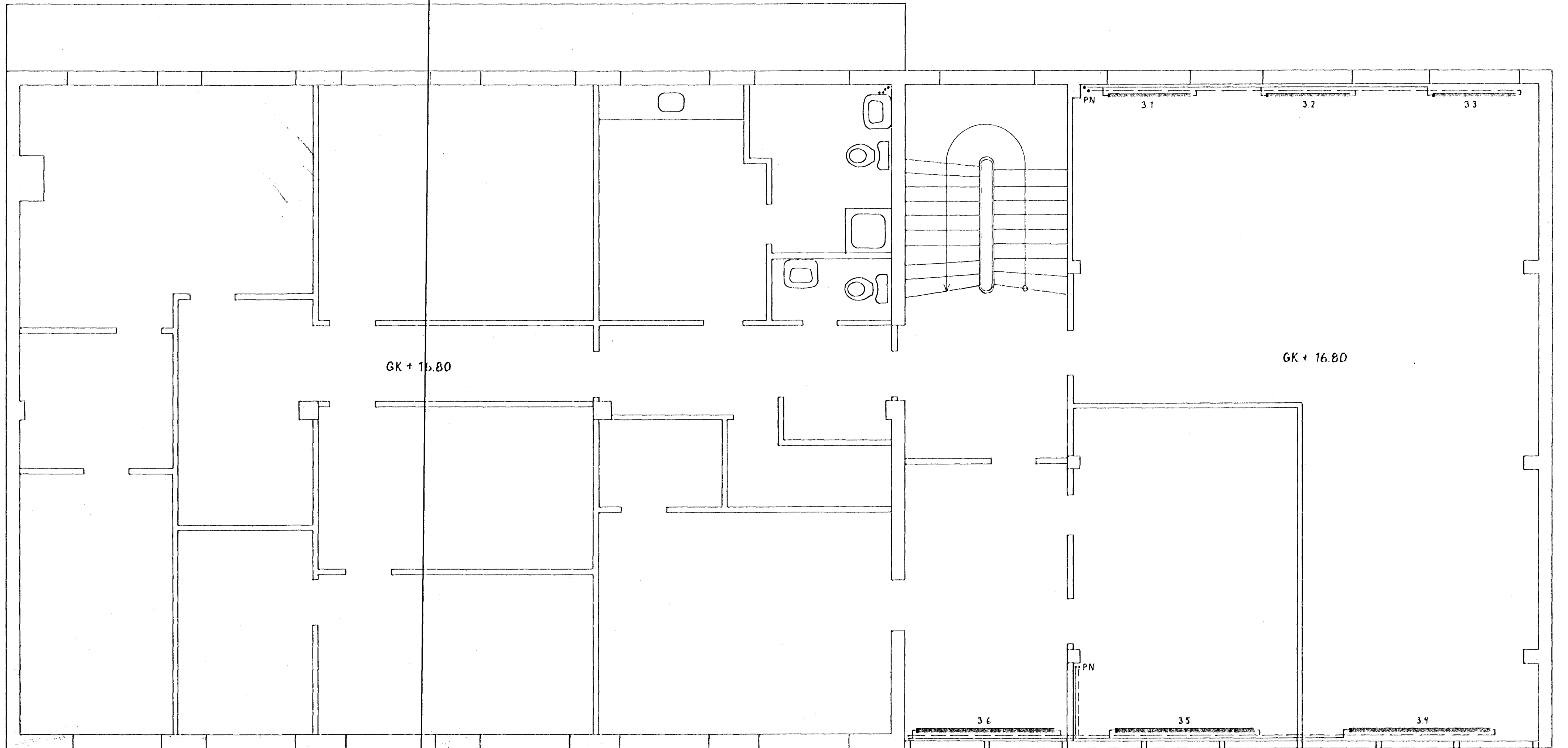
GRUNNMYND 3. HÆÐAR 1:50
