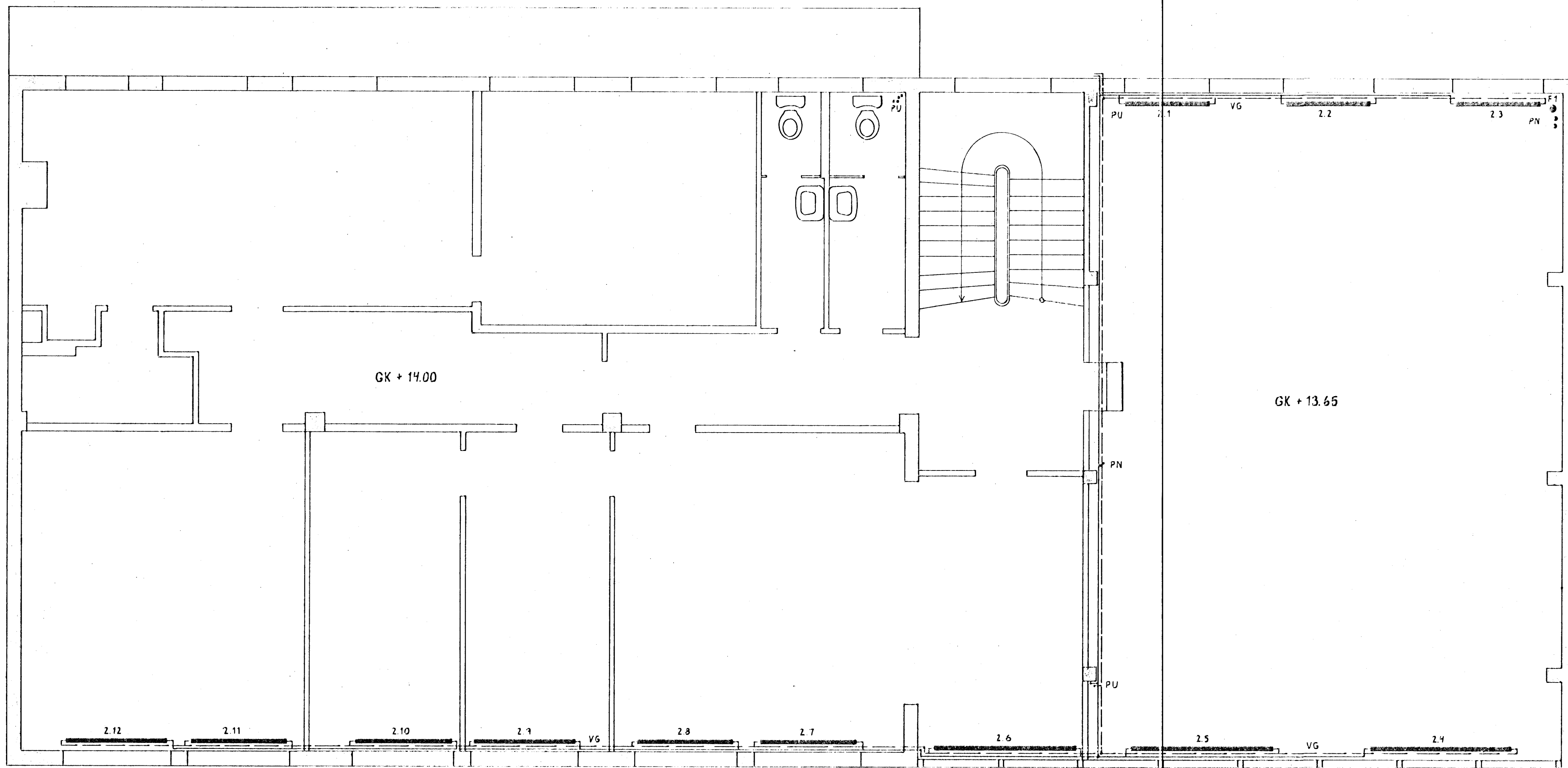
GRUNNMYND 2. HÆÐAR 1:50
