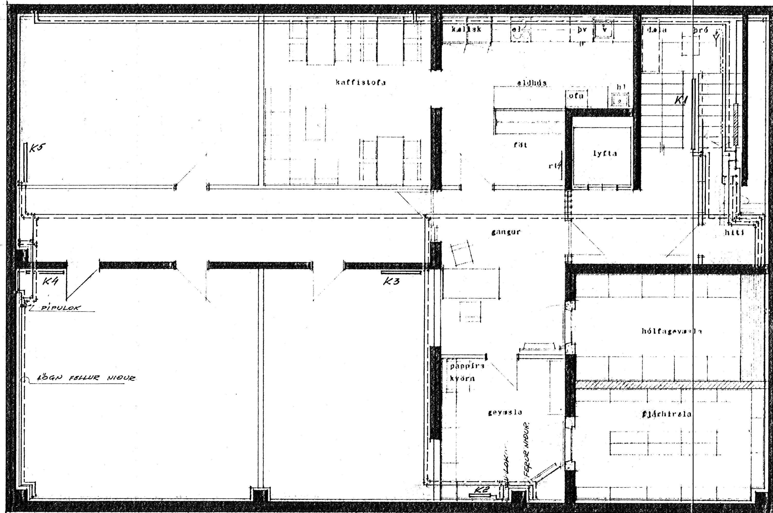
grunnmynd kjallara
