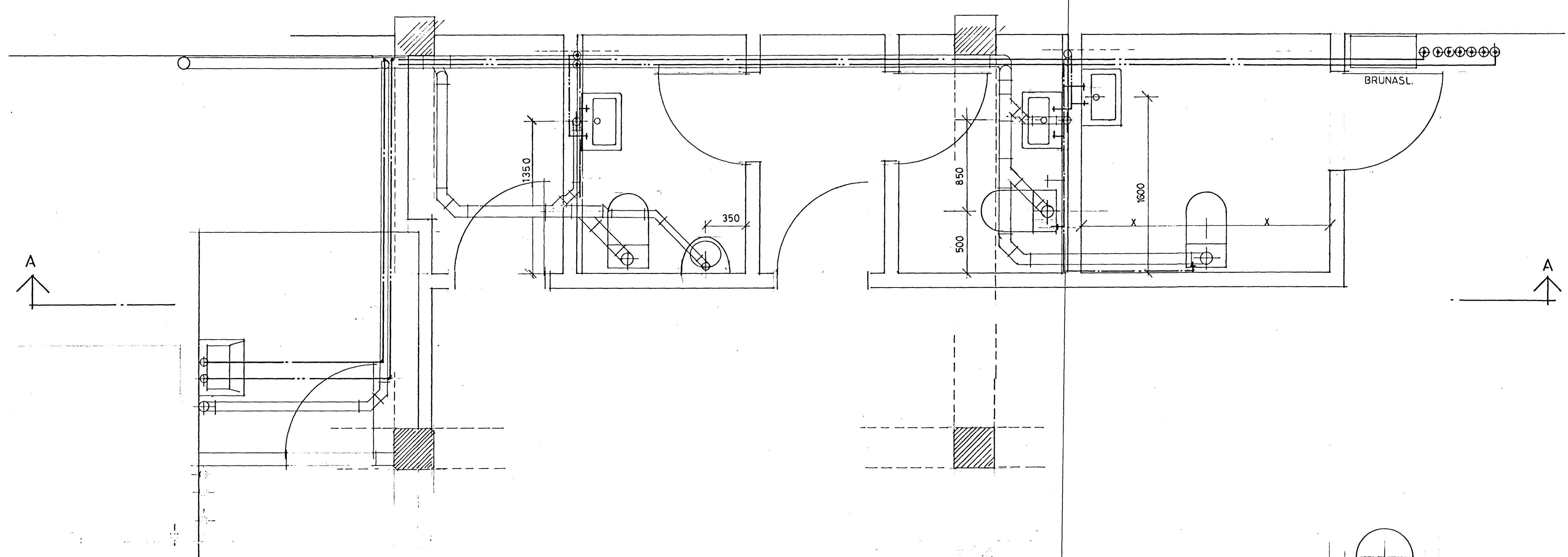
GRUNNMYND 1:20
