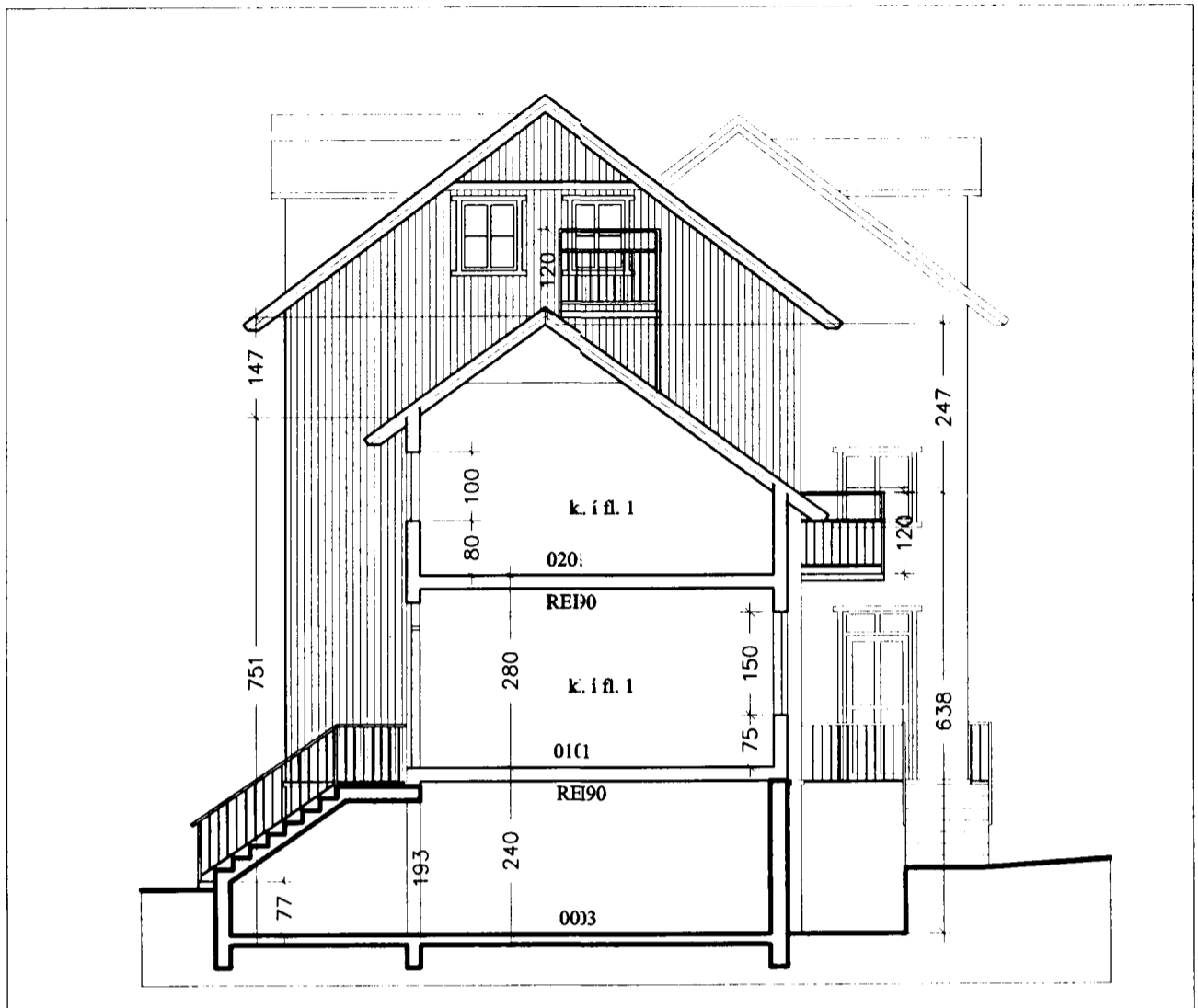
Sneiðing b-b 1:100
