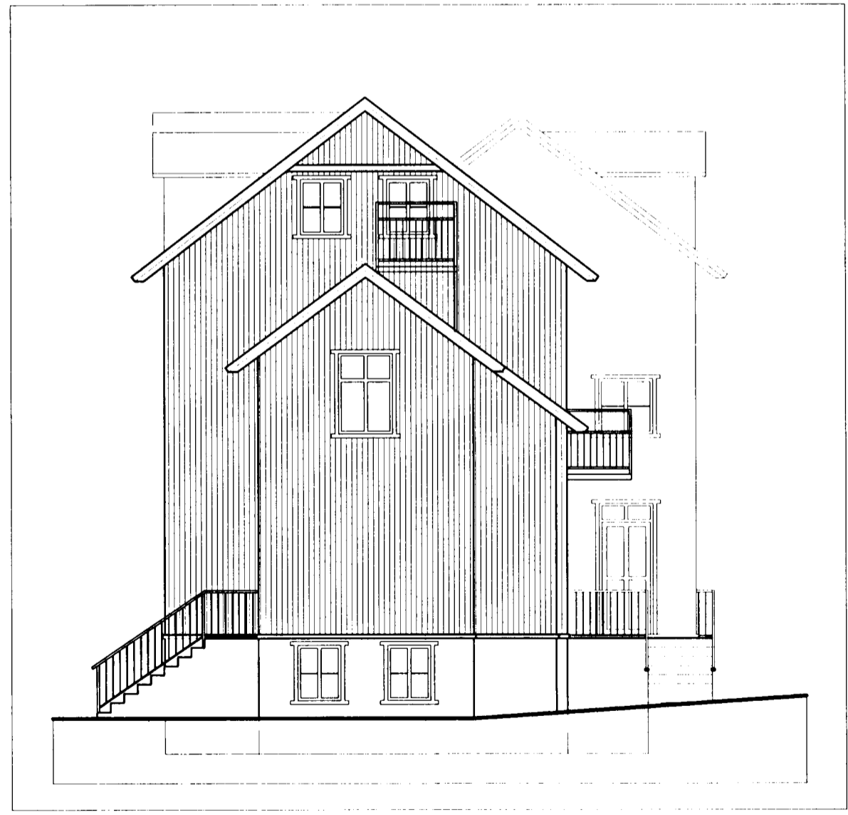
Útlit Austur 1:100
