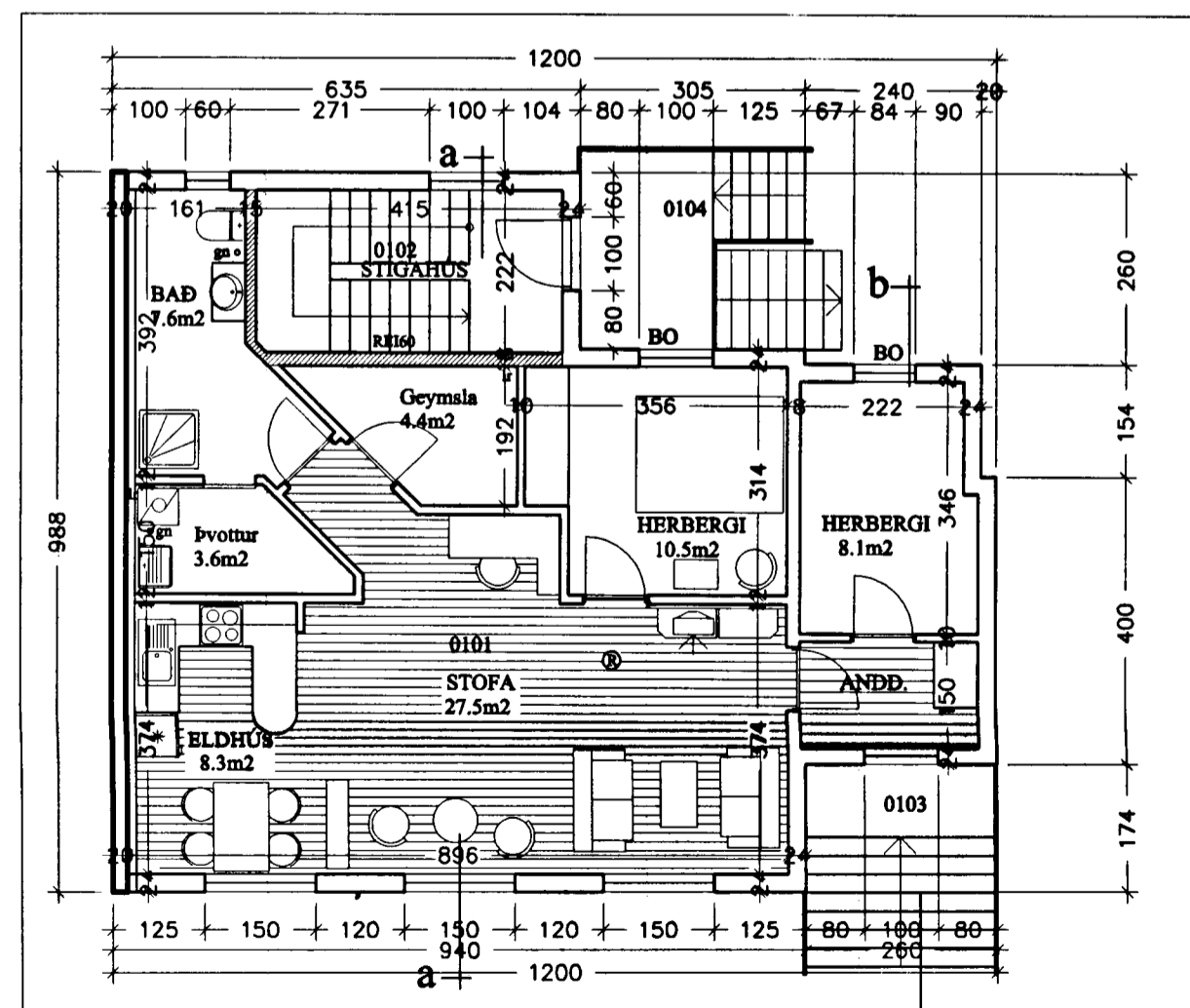
Grunnmynd 1.hæð 1:100
