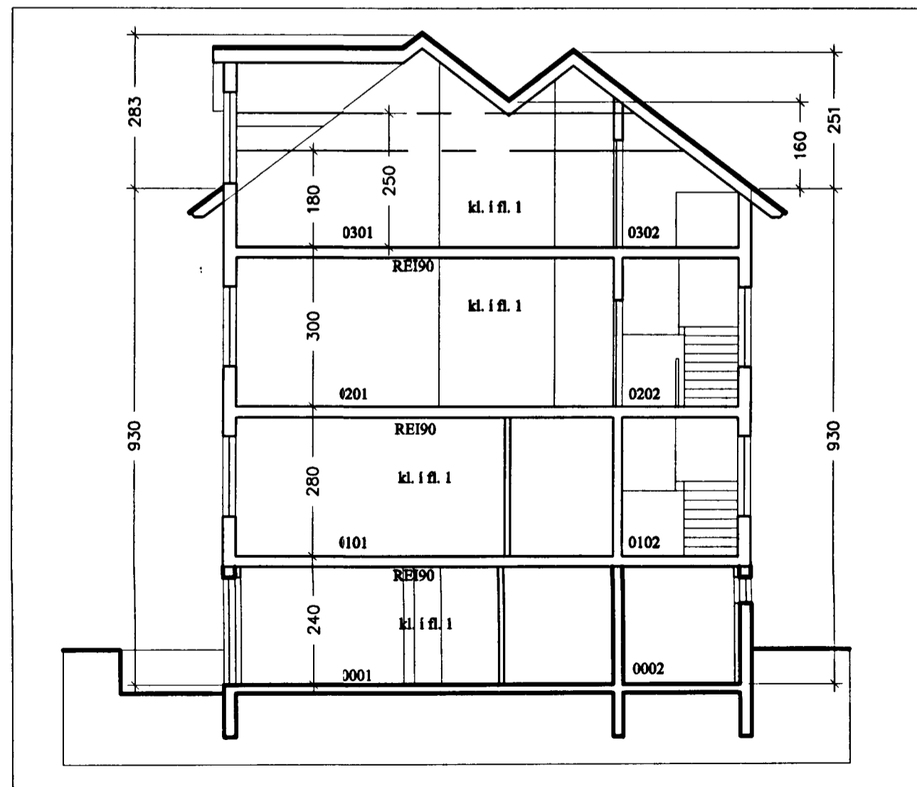
Sneiðing a-a 1:100
