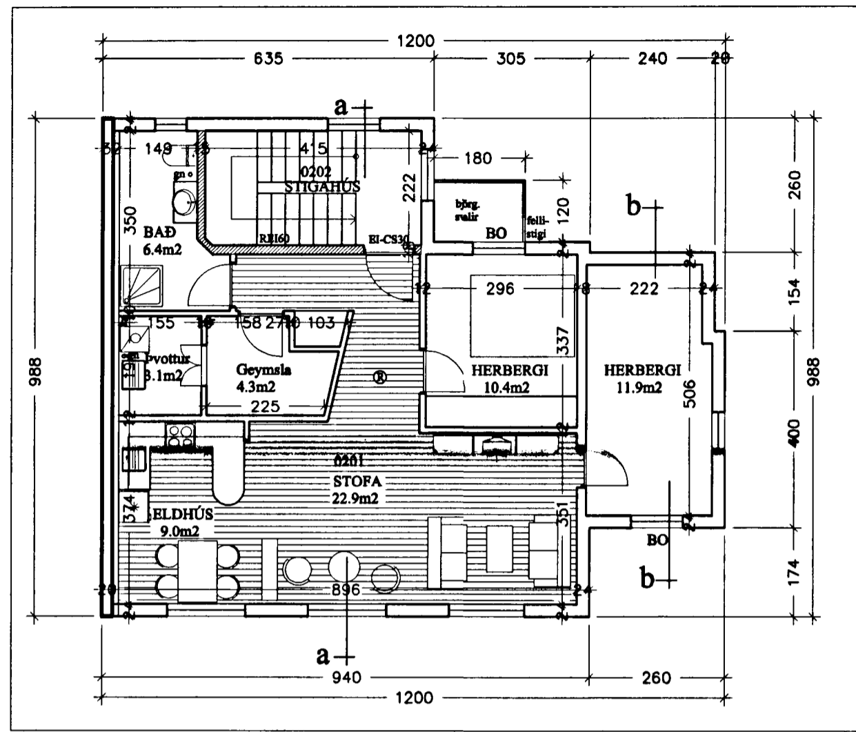
Grunnmynd 2.hæð 1:100
