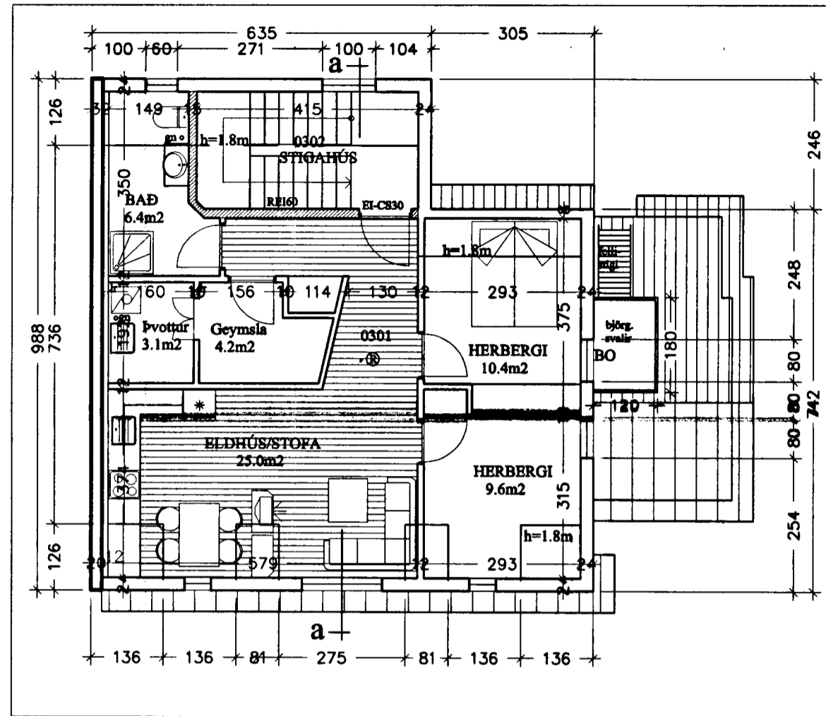
Grunnmynd 1.hæð 1:100
