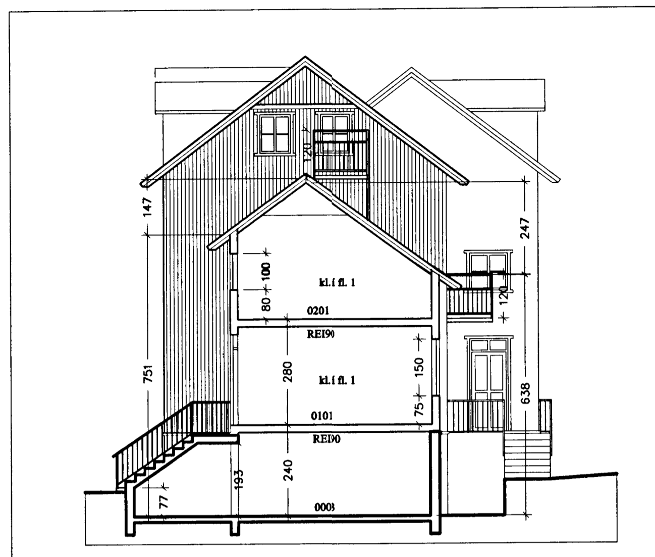
Sneiðing b-b 1:100
