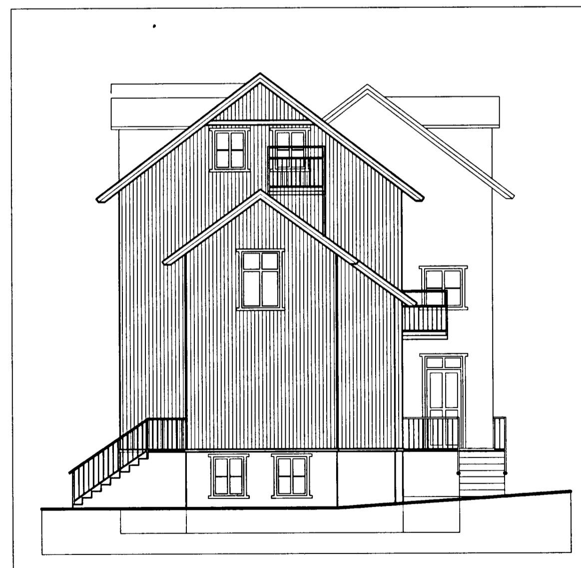
Útlit Austur 1:100
