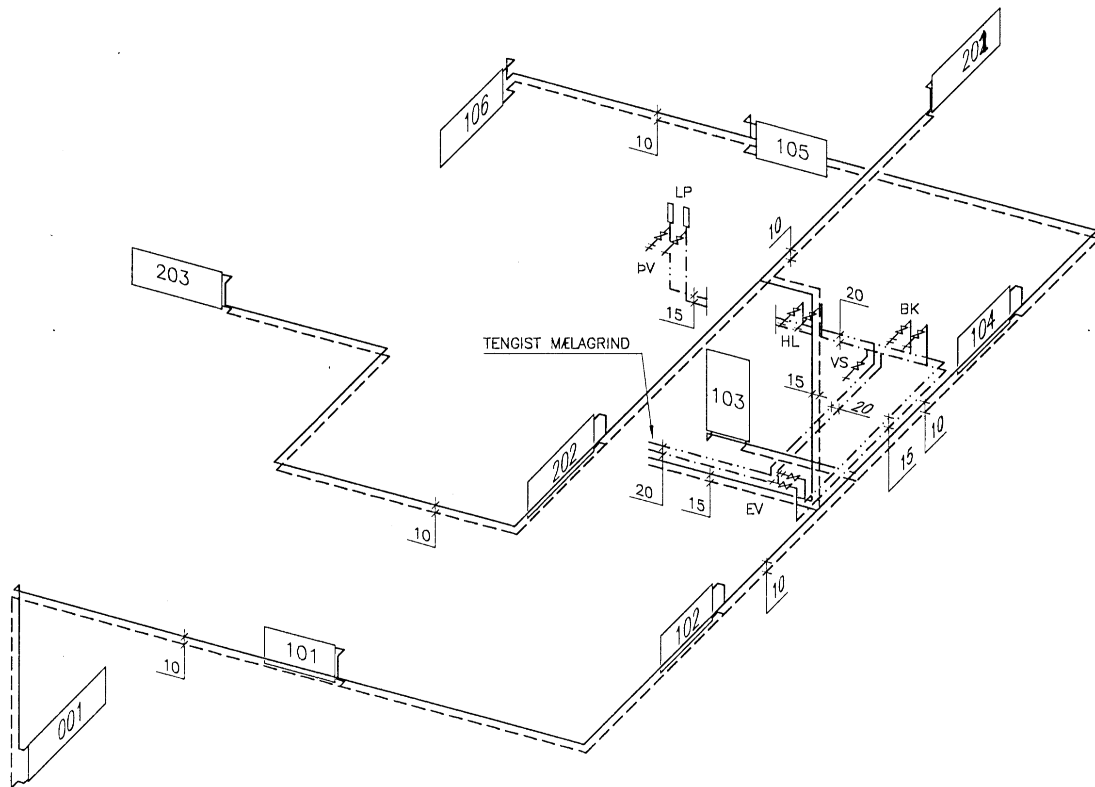
RÚMMYND 1:50
