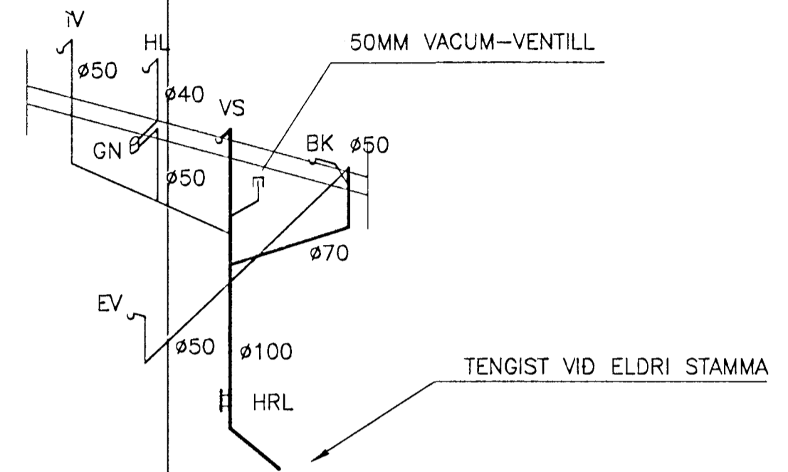
SKOLPSTAMMI F1 1:50
