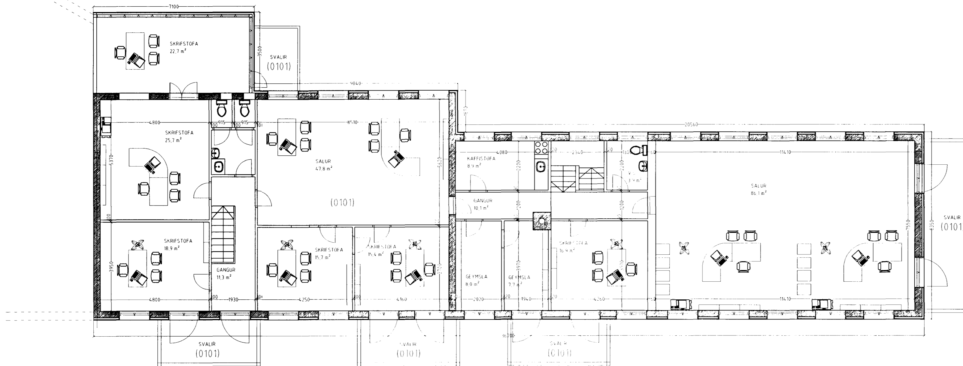
Grunnmynd 2. hæð m.kv. 1:100.
