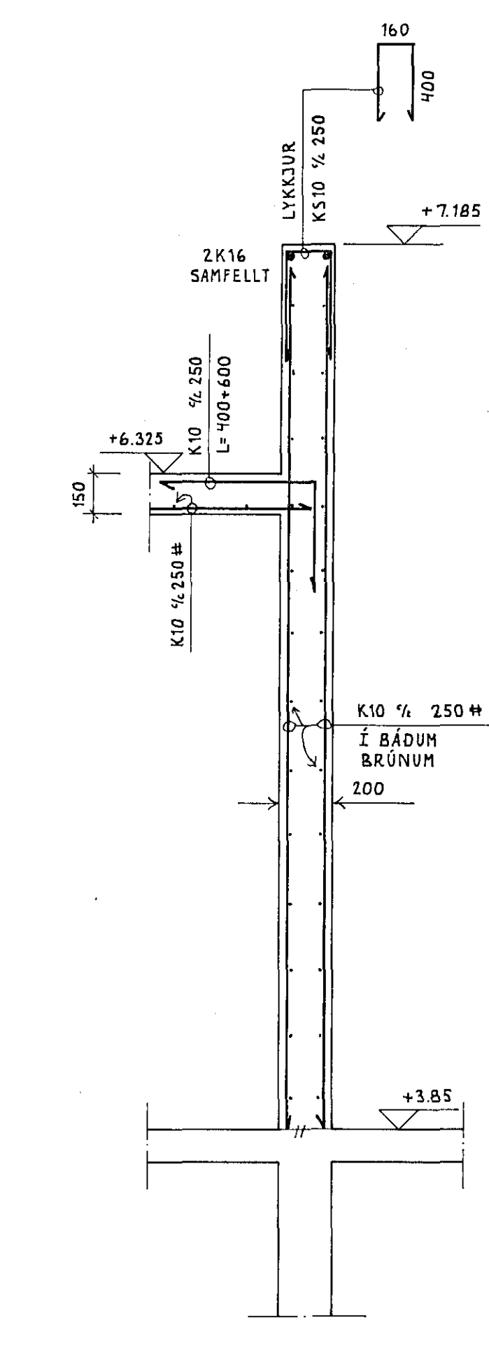
SNID A-A 1:20
