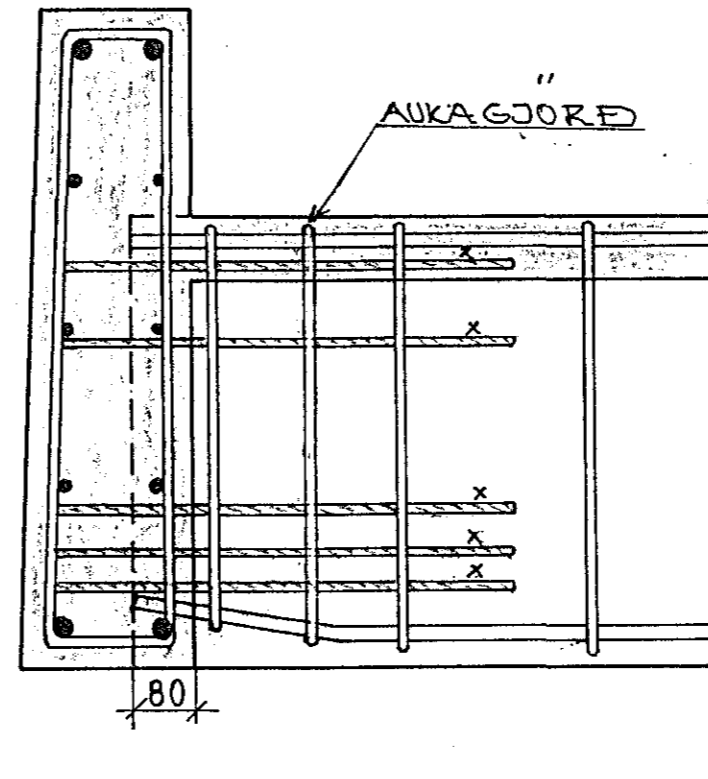
SNID B-B 1:10
