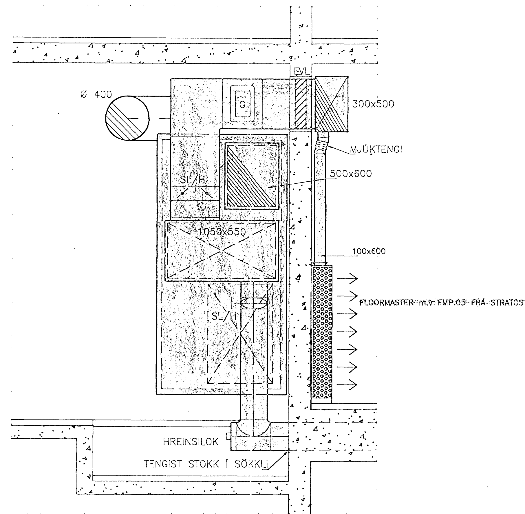
1 Snið M. 1:20
