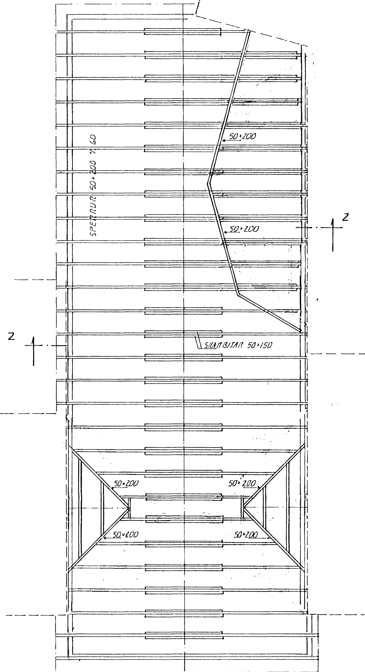
GRUNNMÝND ÞAK. 1:50
