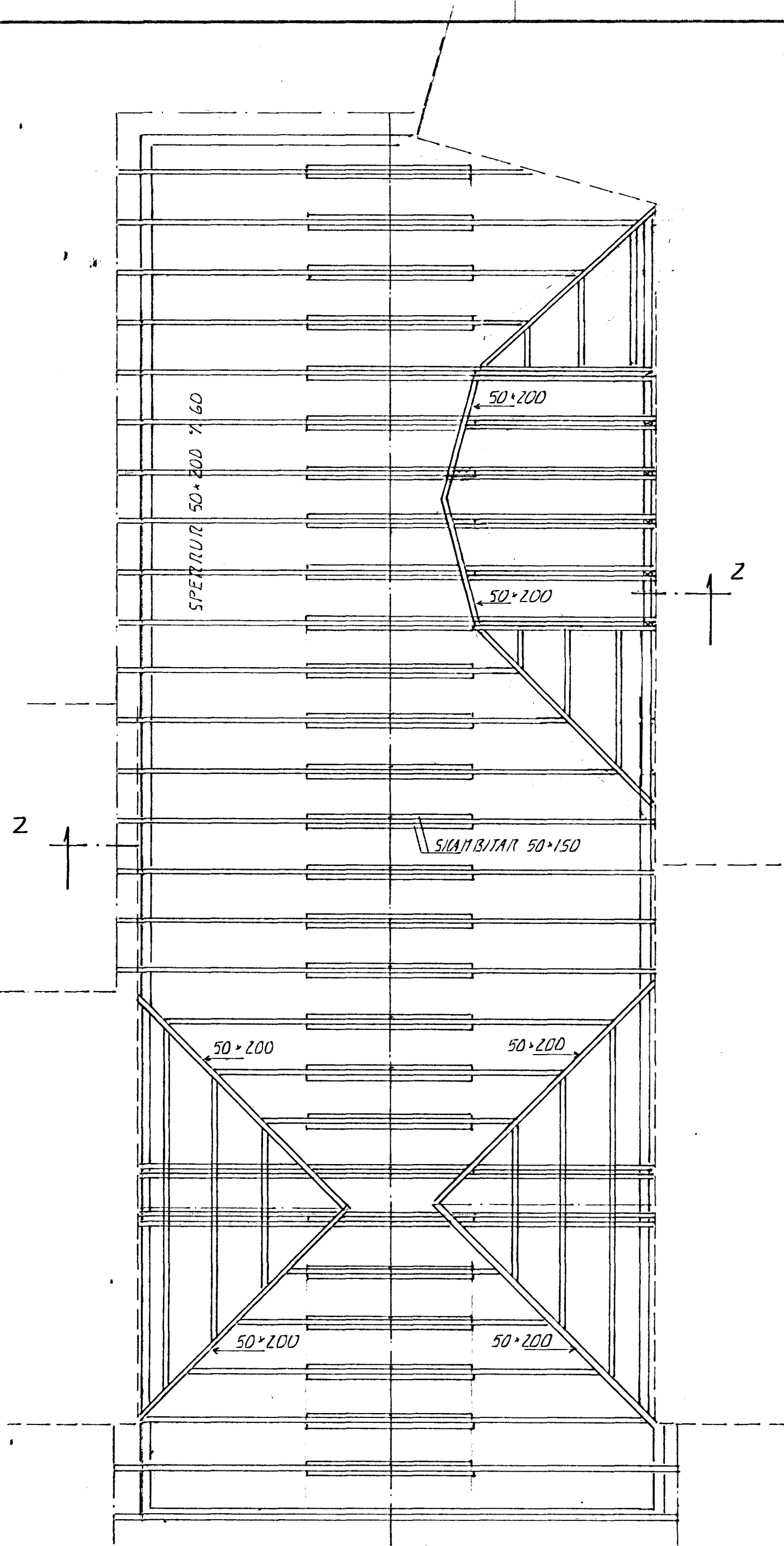
GRUNNMÝND BAK. 1:50
