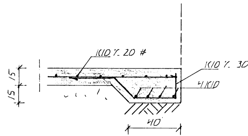
SNID 1. 1:20
