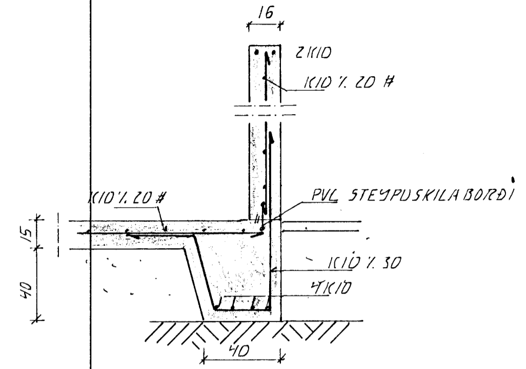
SNID 4. 1:20
