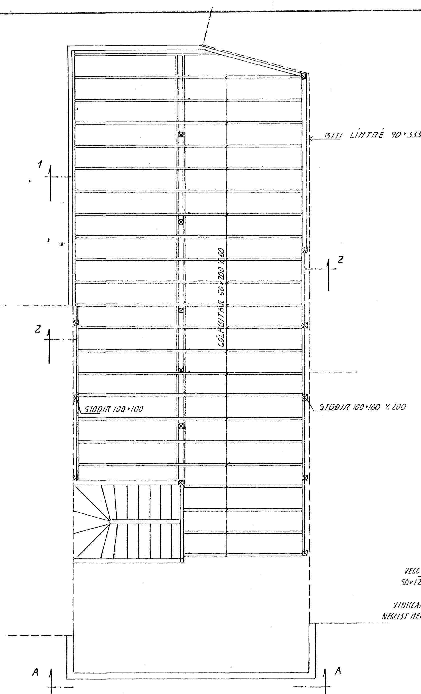
GRUNNMÝND MILLIGÓLF. 1:50
