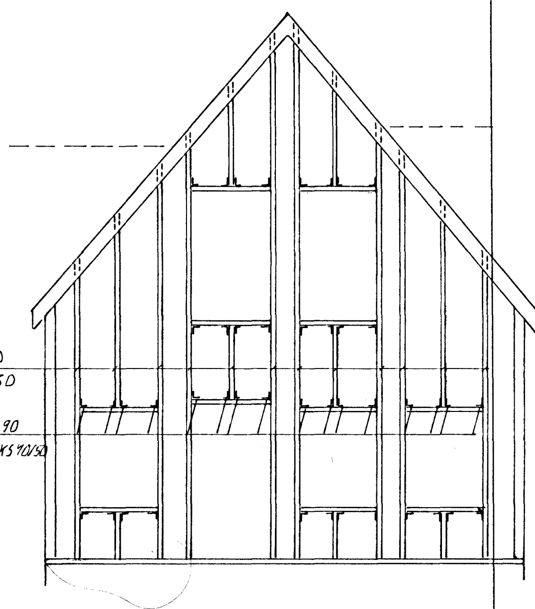
ÁSYND A-A GAFL. 1:50
