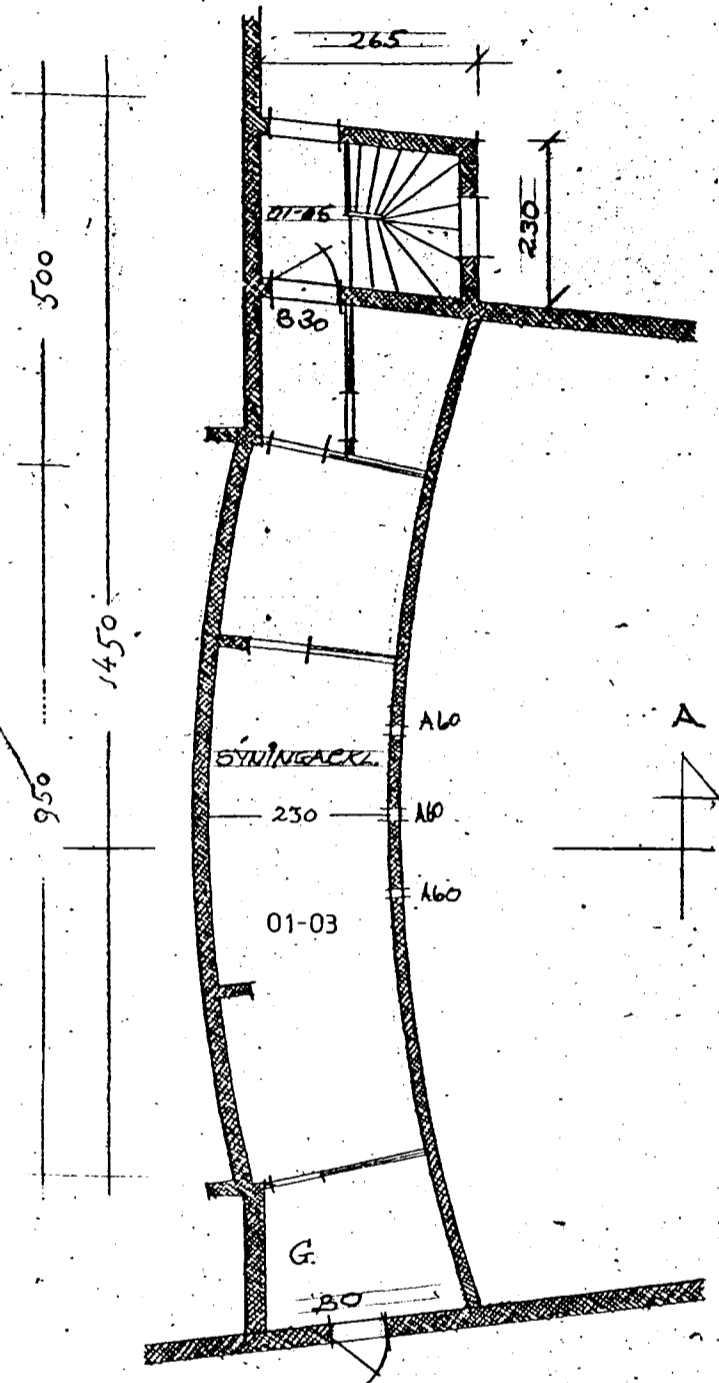
GRUNNMYND MÍLLÍDFTS MKV: 1:100
