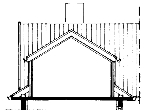
SNEIÐING Í KVIST Í STOFU 1:100
