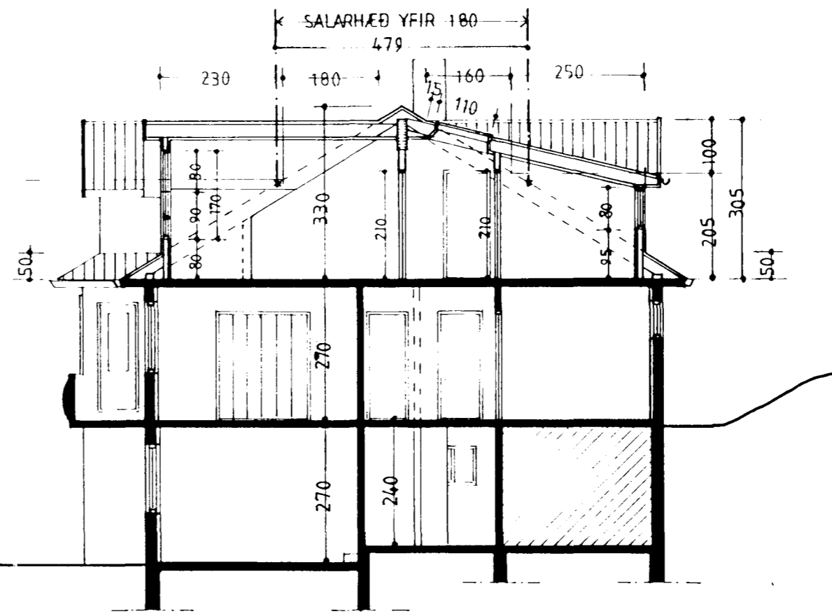
SNEIÐING A-A 1:100
