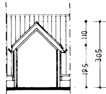
SNEIÐING Í KVIST Í BORÐSTOFU (OG VINNUHERB.) 1:100
