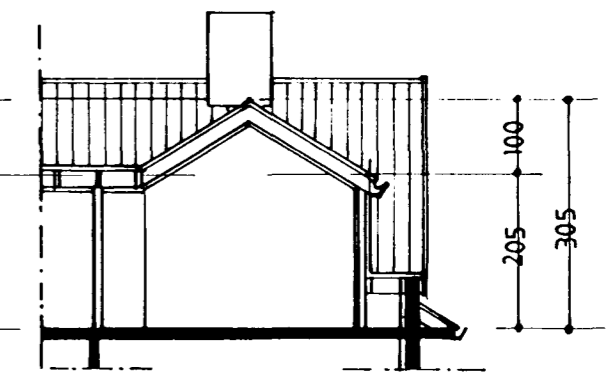
SNEIÐING Í KVIST Í SVEFNHERBERGI (OG ELDHÚSI) 1:100
