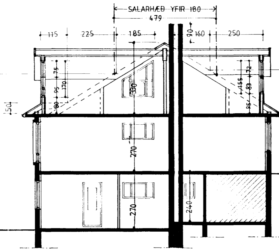
SNEIÐING B-B 1:100
