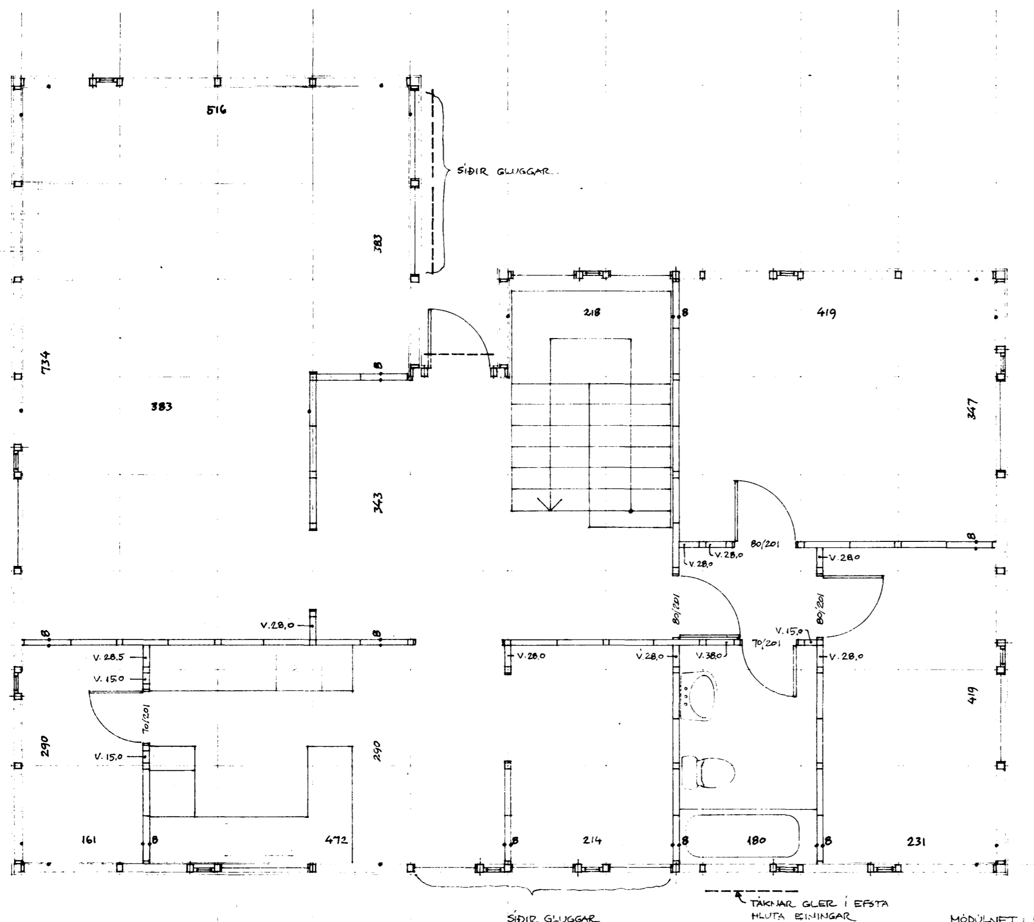
GRUNNMYND, 1:50
