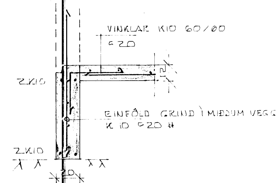
SNID I ÚTV. 1:20
