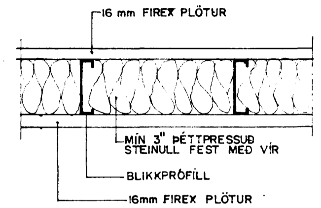
HLUTAMYND AF B-60 VEGG. M:1:5
