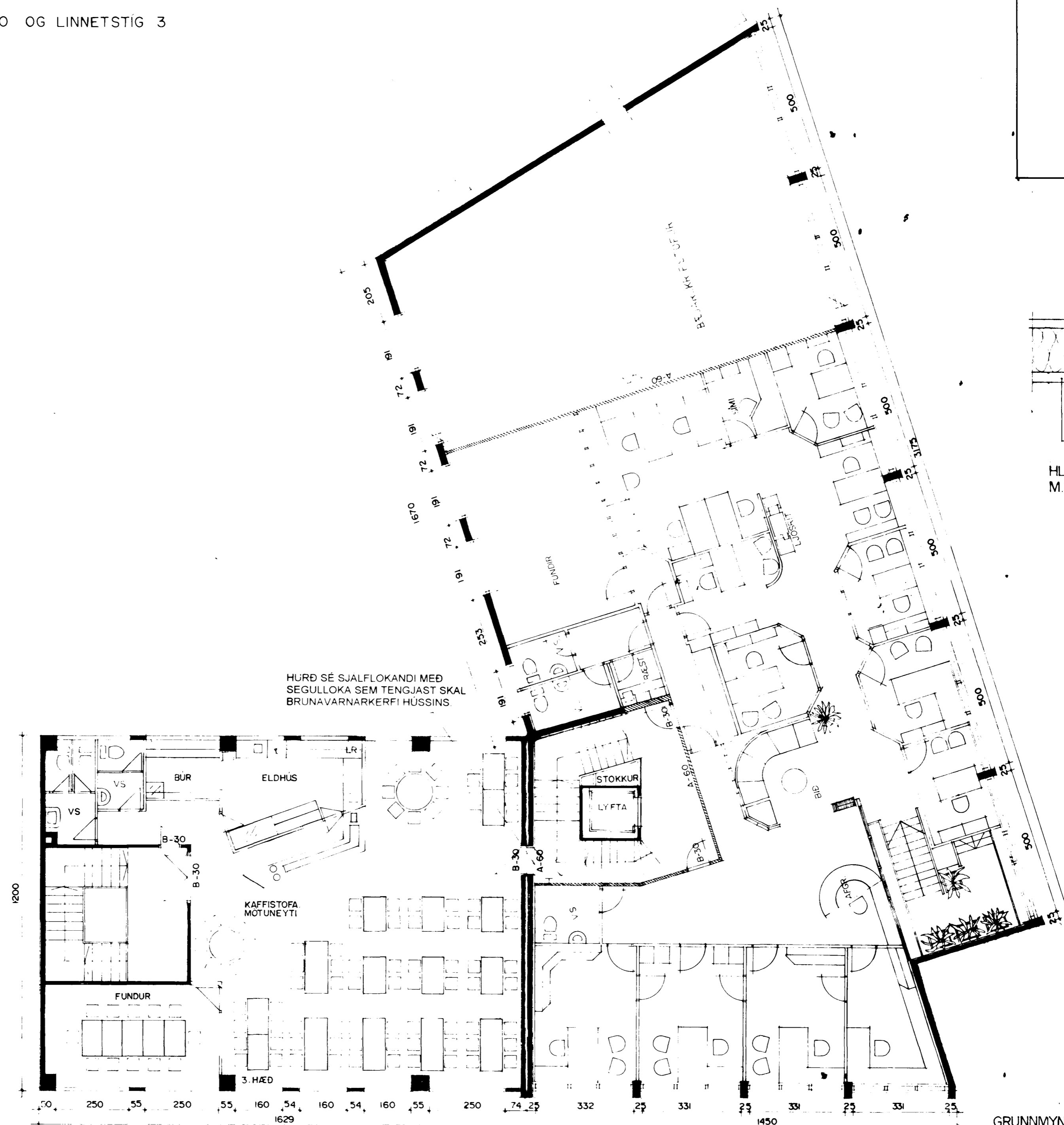
GRUNNMYND 3 HÆÐAR LINNETSTÍGS 3 MKV. 1 : 100
