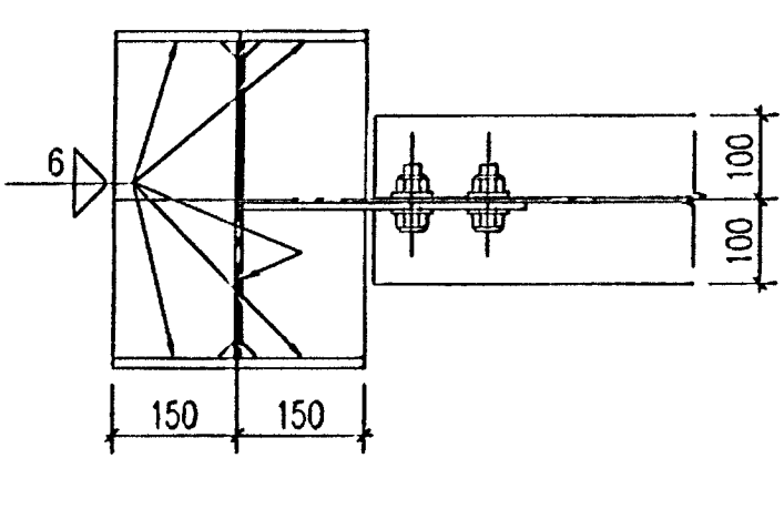
C--C Scale 1:10
