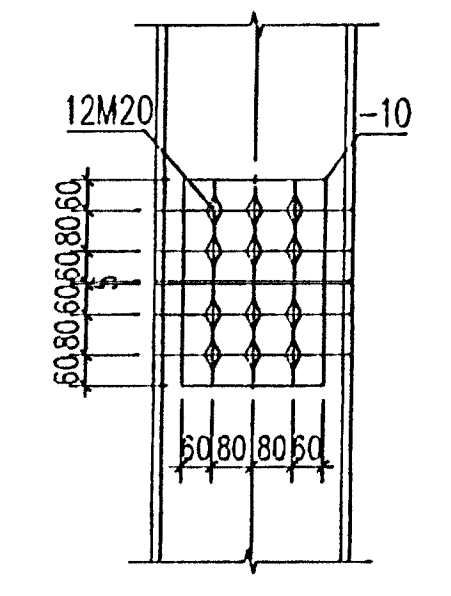
A--A Scale 1:15
