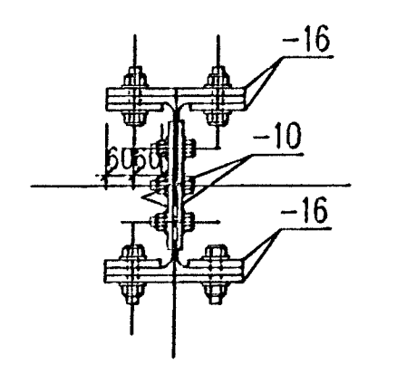
B--B Scale 1:15
