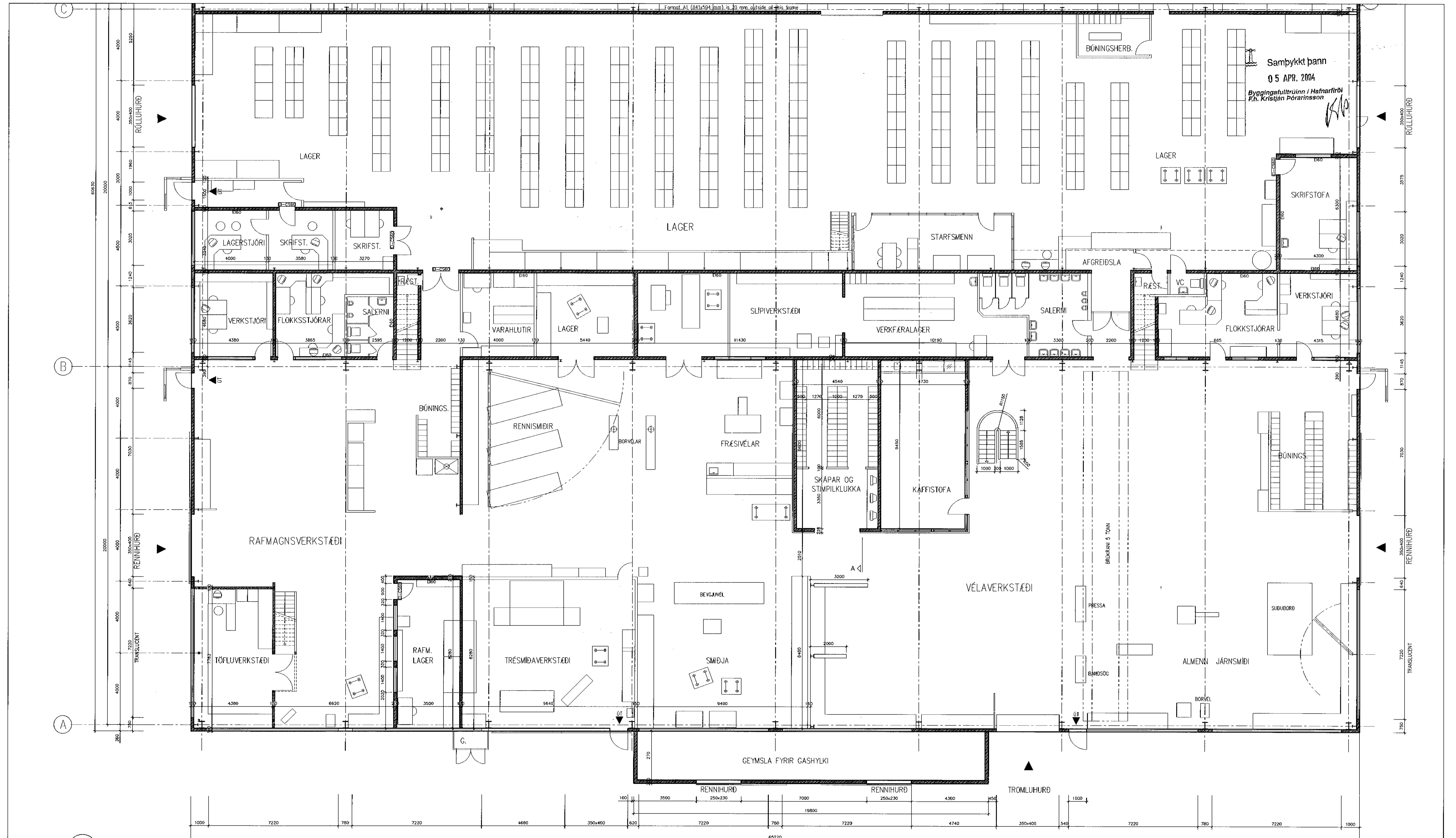
GRUNNMYND 1.HÆÐ MKV.1:100
