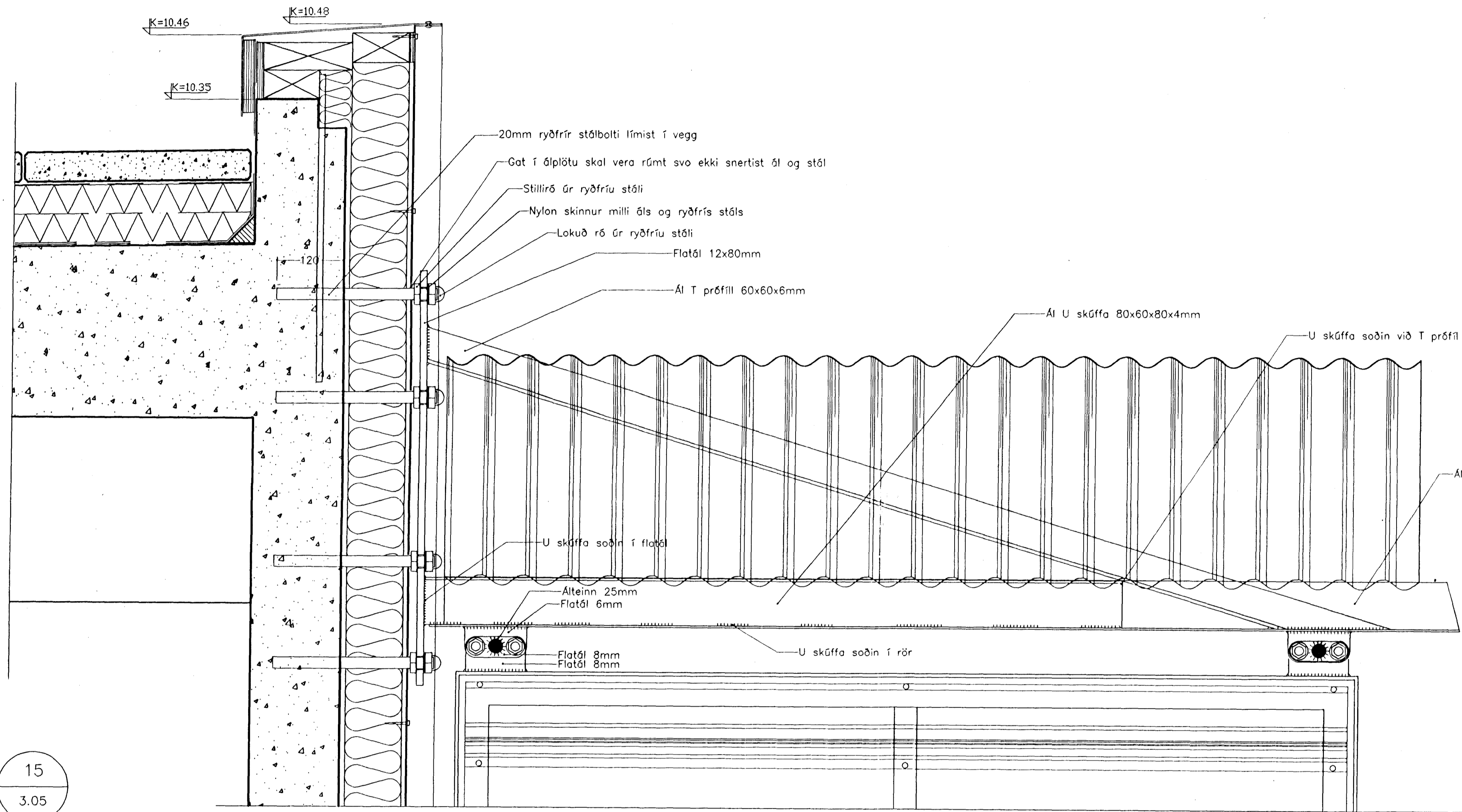
LÓDRÉTT SNID FESTING FYRIR SKYGGNI VID VEGG 1:5
