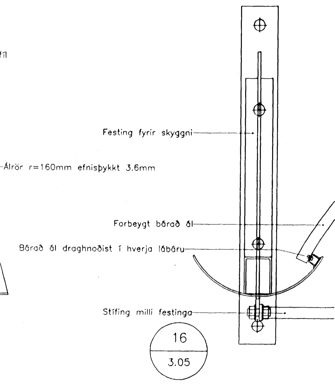
ASÝND FRAMAN Á FESTINGU 1:5
