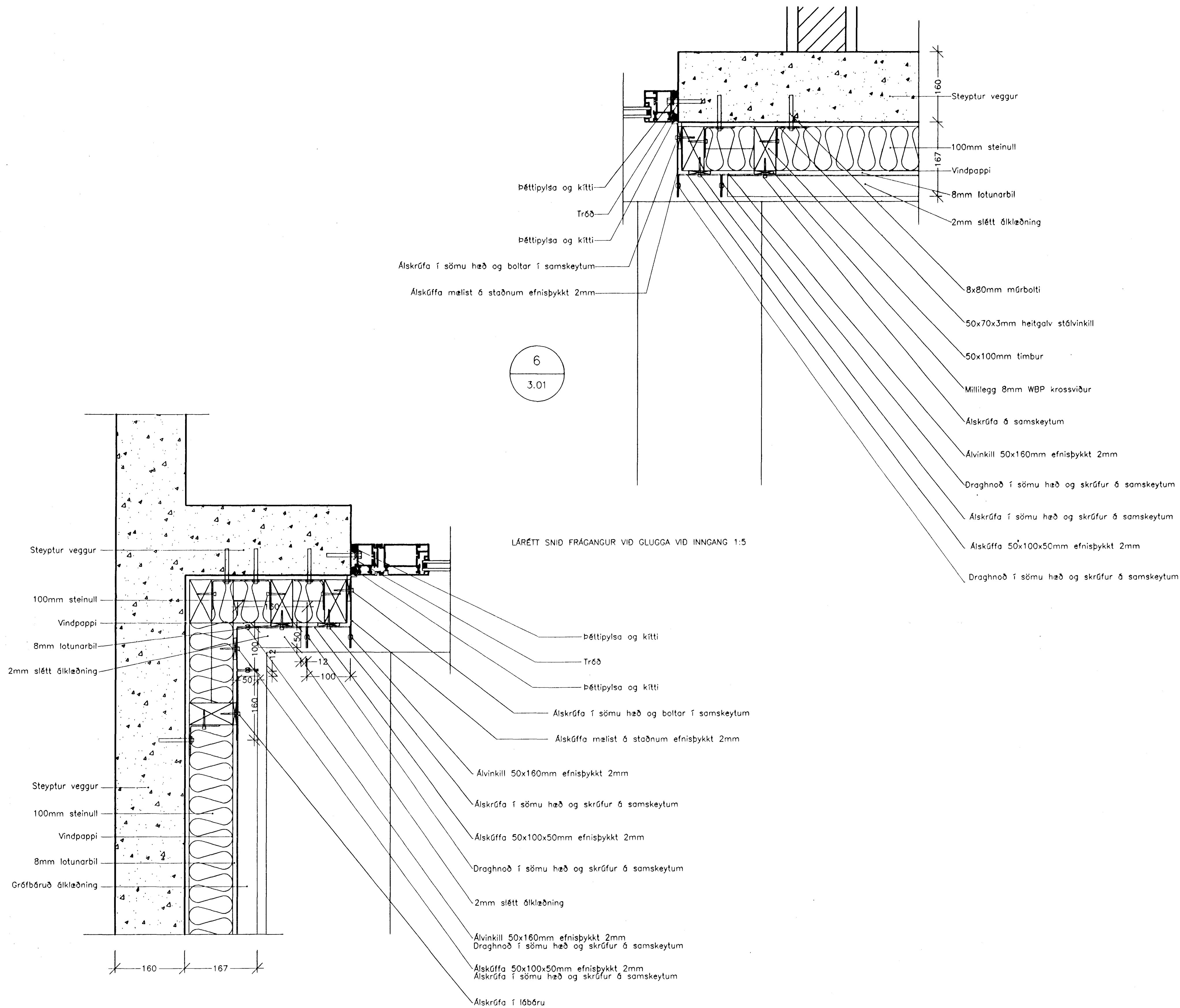
LÁRÉTT SNID FRÁGANGUR VID INNGANG 1:5
