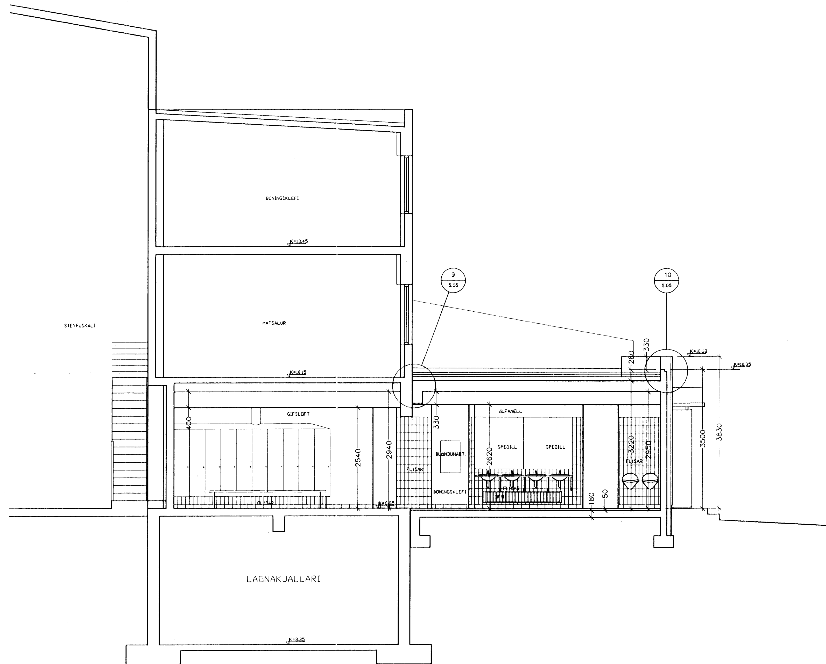
SNEIDING A-A 1:50
