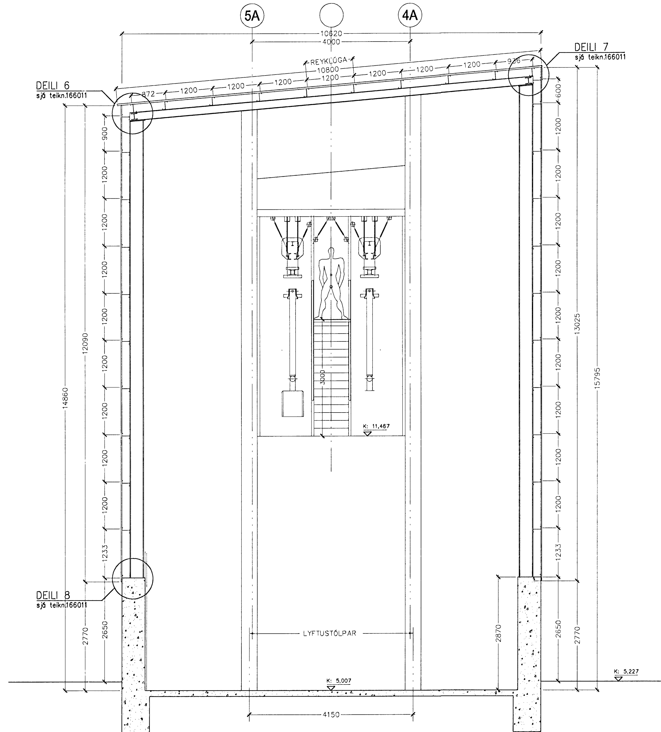
SNEIÐING B-B
