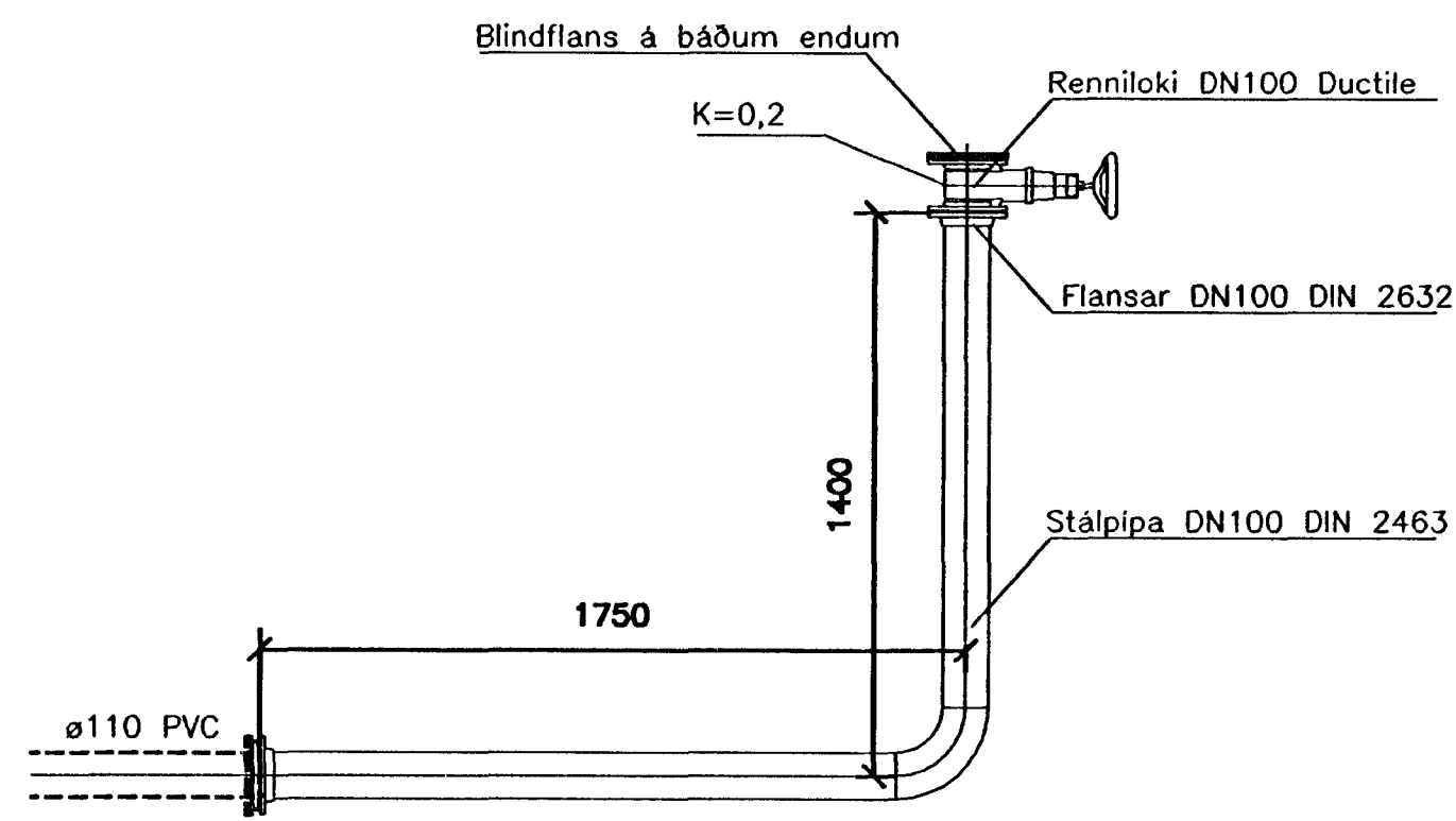
Vatnsinntak M. 1:20
