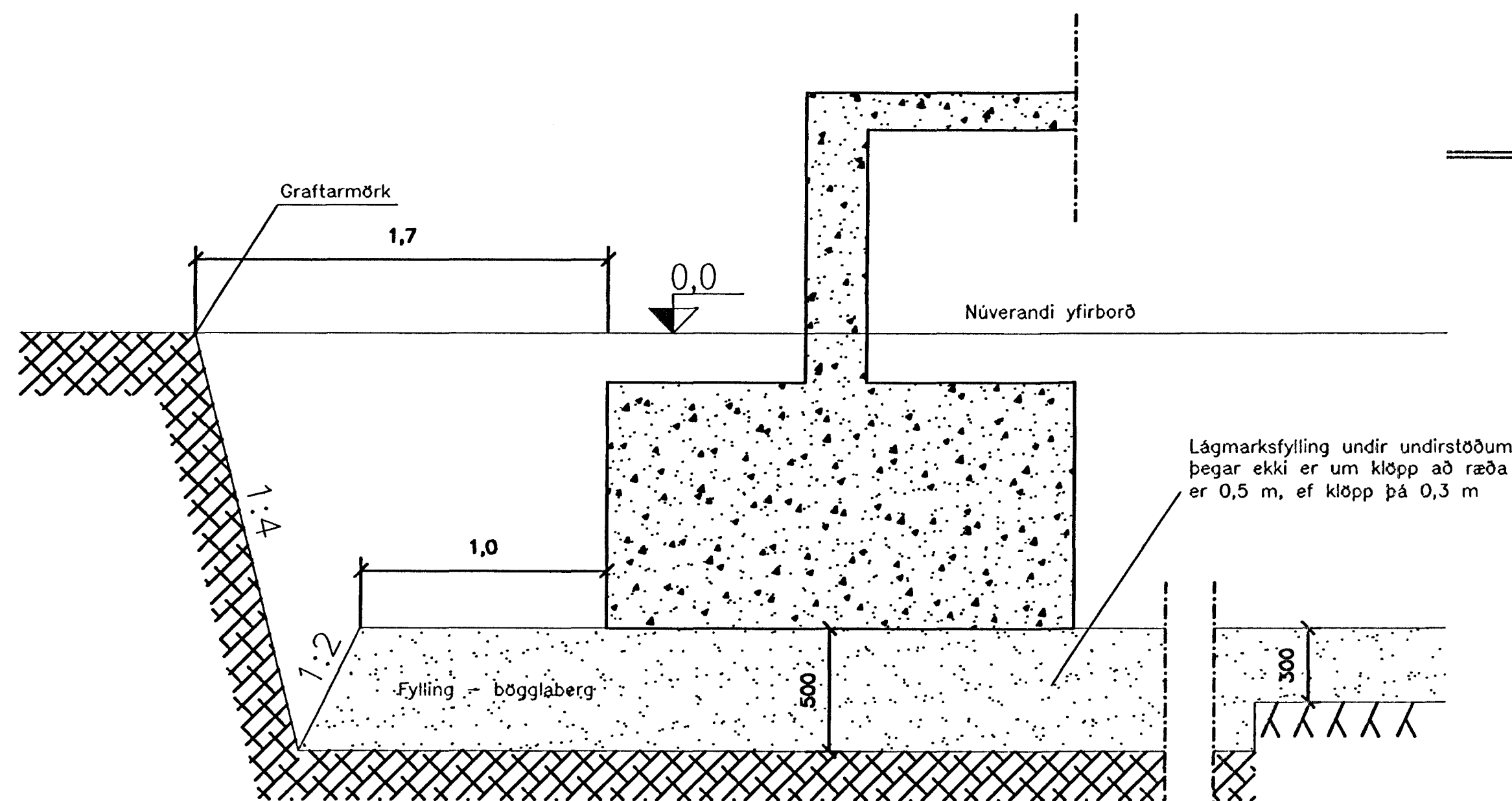
Snið A-A Graftarmörk, kennisnið M. 1:20
