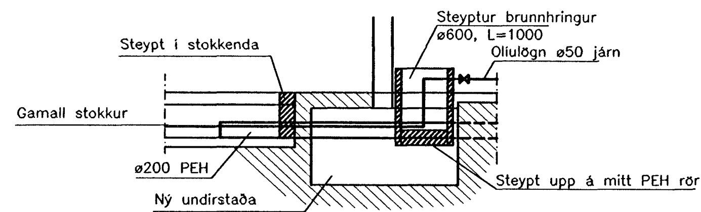
Snið B-B Inntök olíulagna M. 1:50
