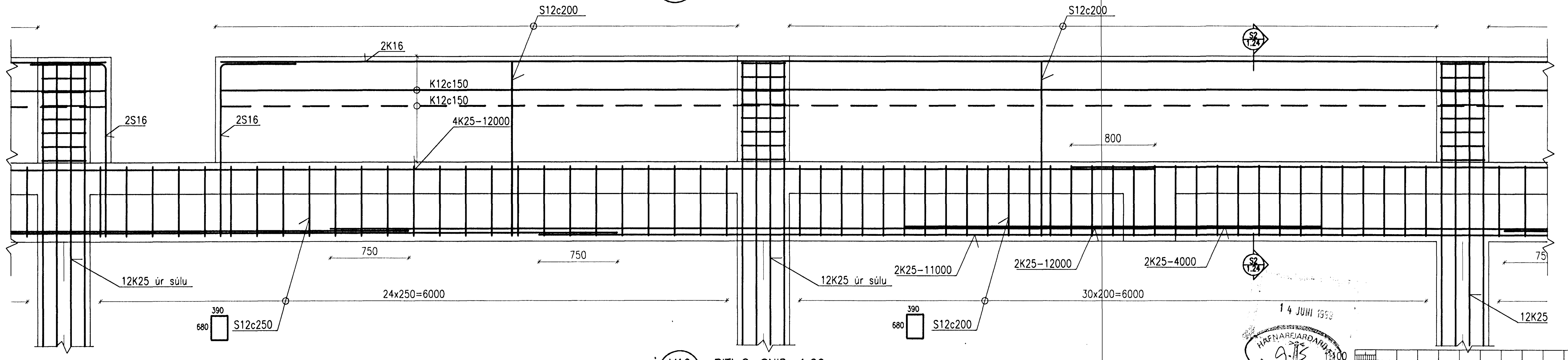
V19 BITI 8, SNID, 1:20
