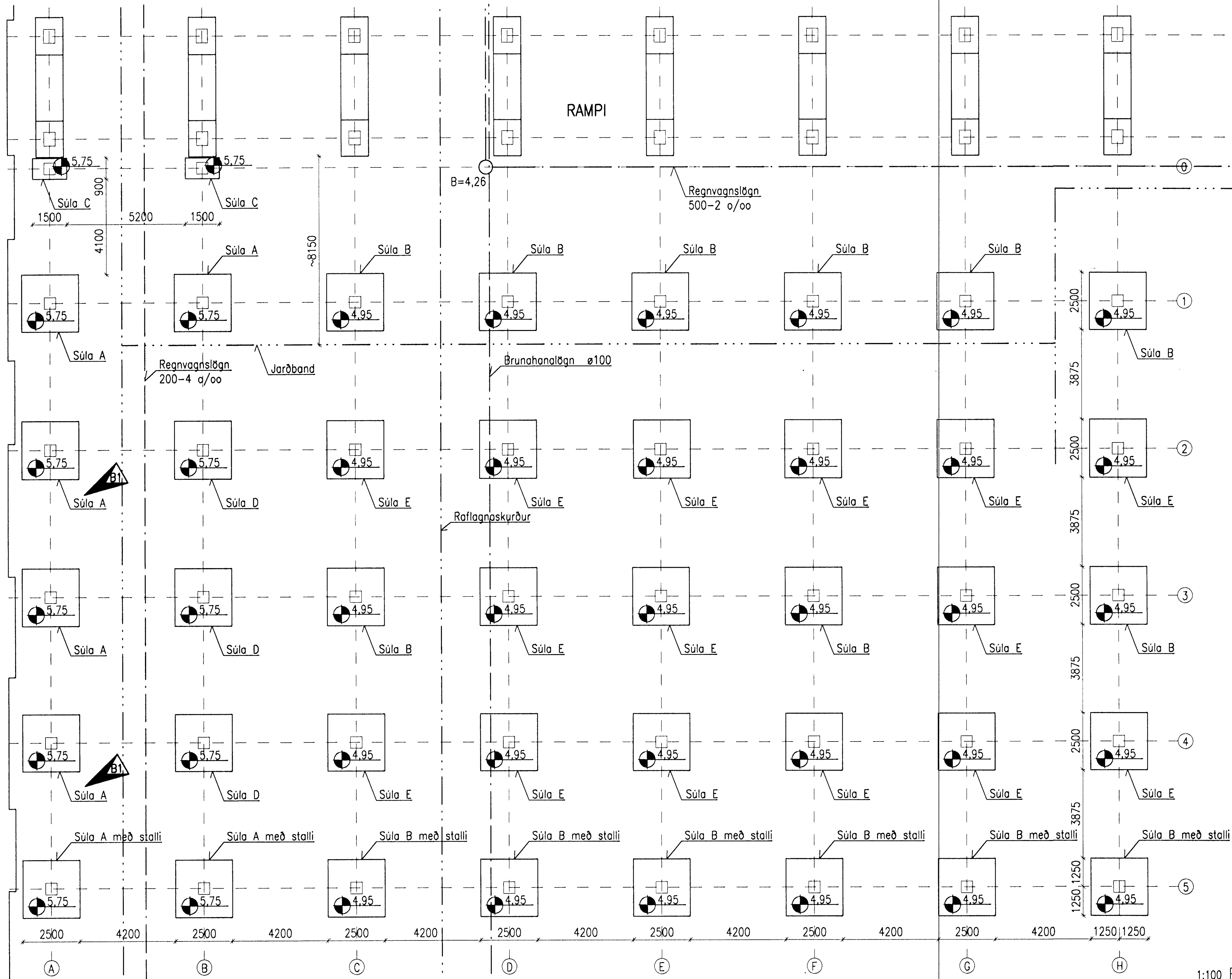
U1 UNDIRSTÖÐUR, PLAN, 1:100
