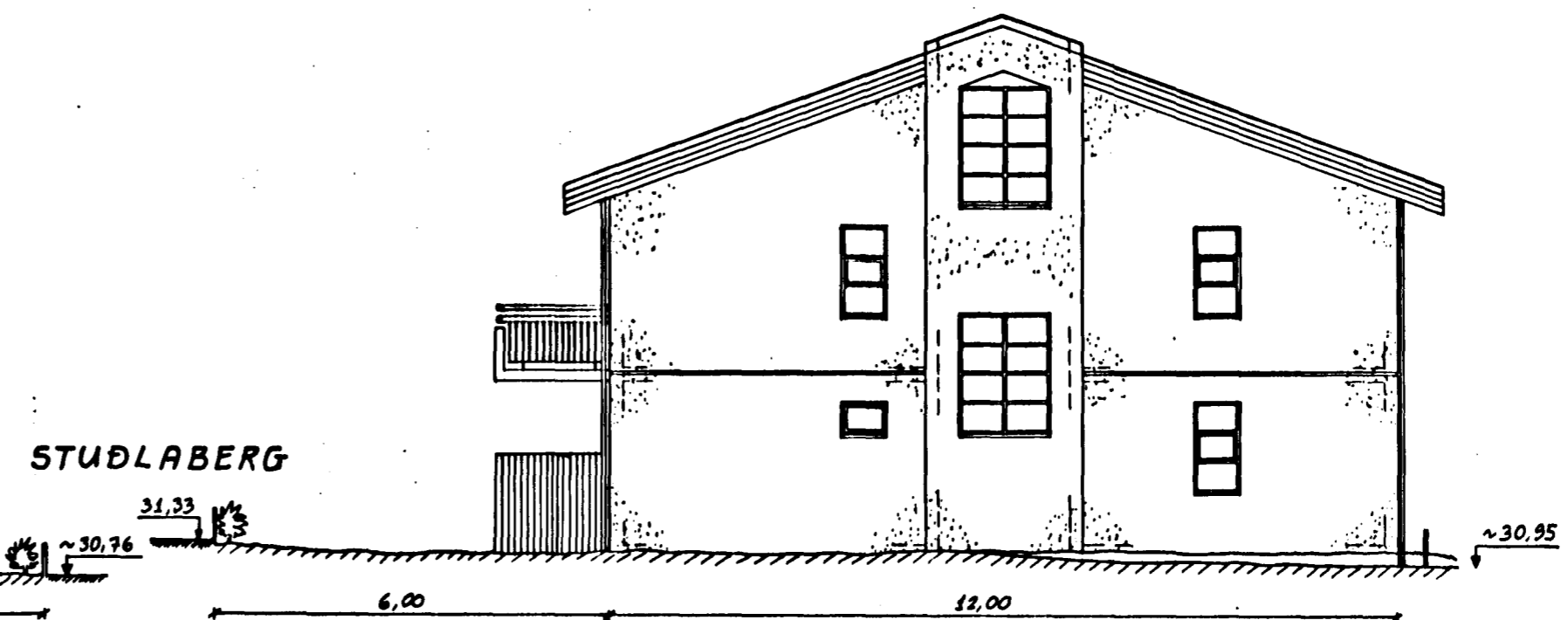
AUSTURHLIÐ. 1:100
