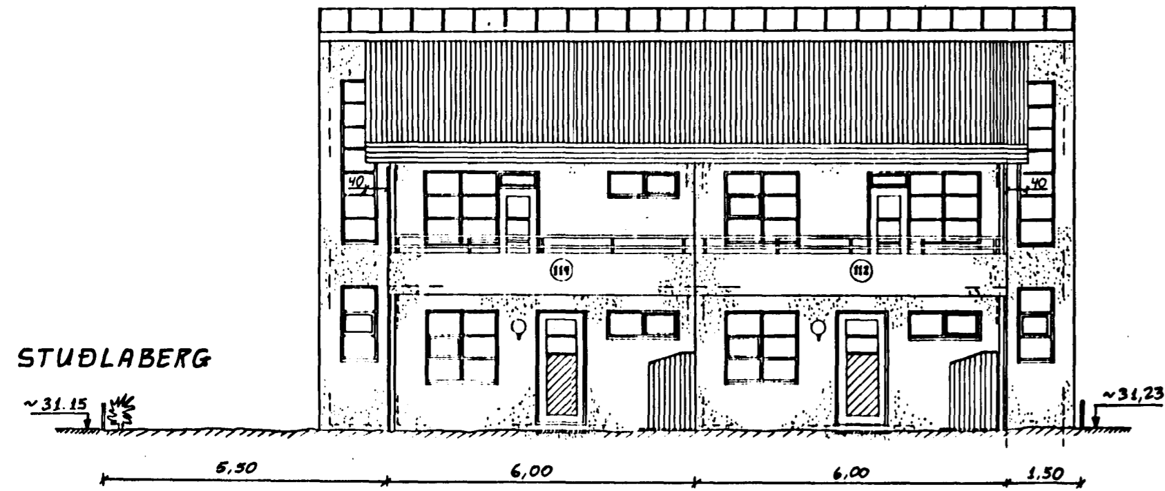
SUDURHLIÐ. 1:100
