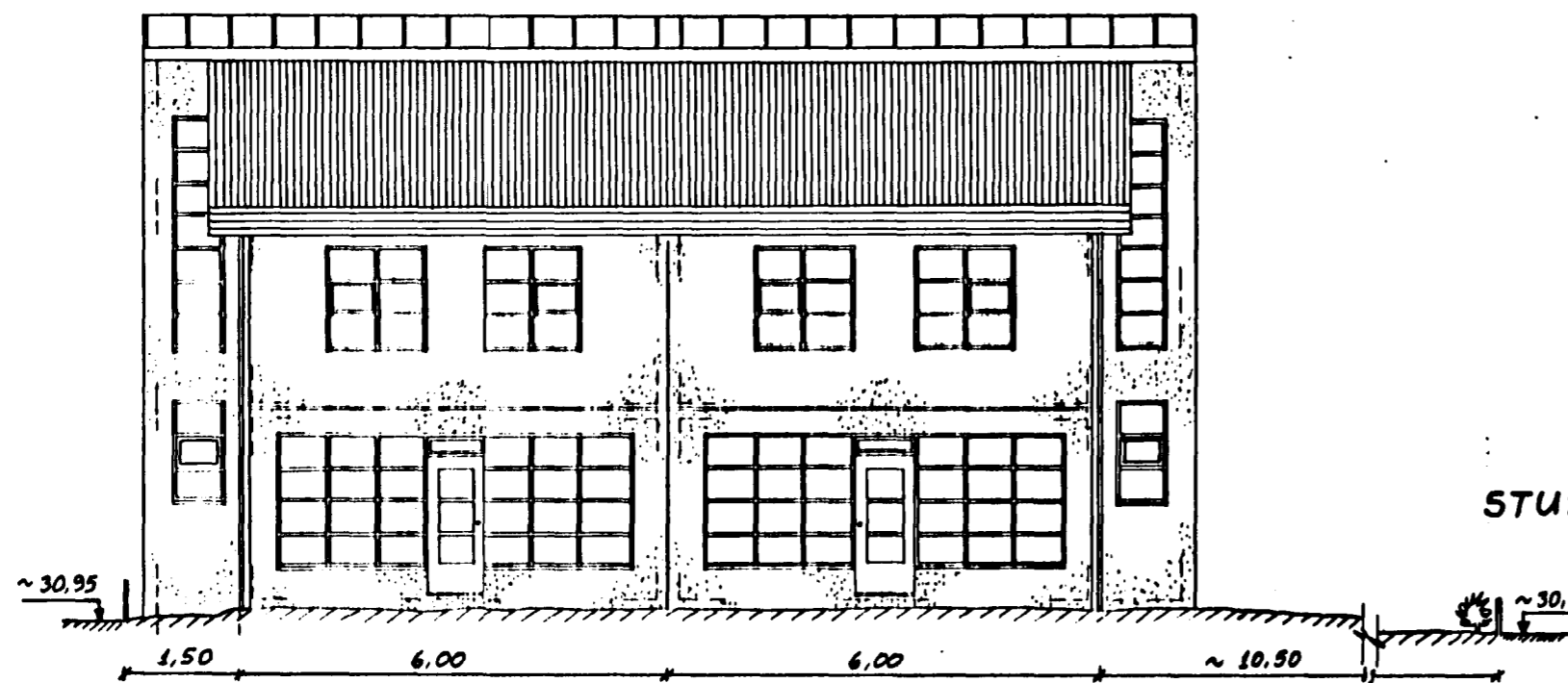
NORDURHLIÐ. 1:100
