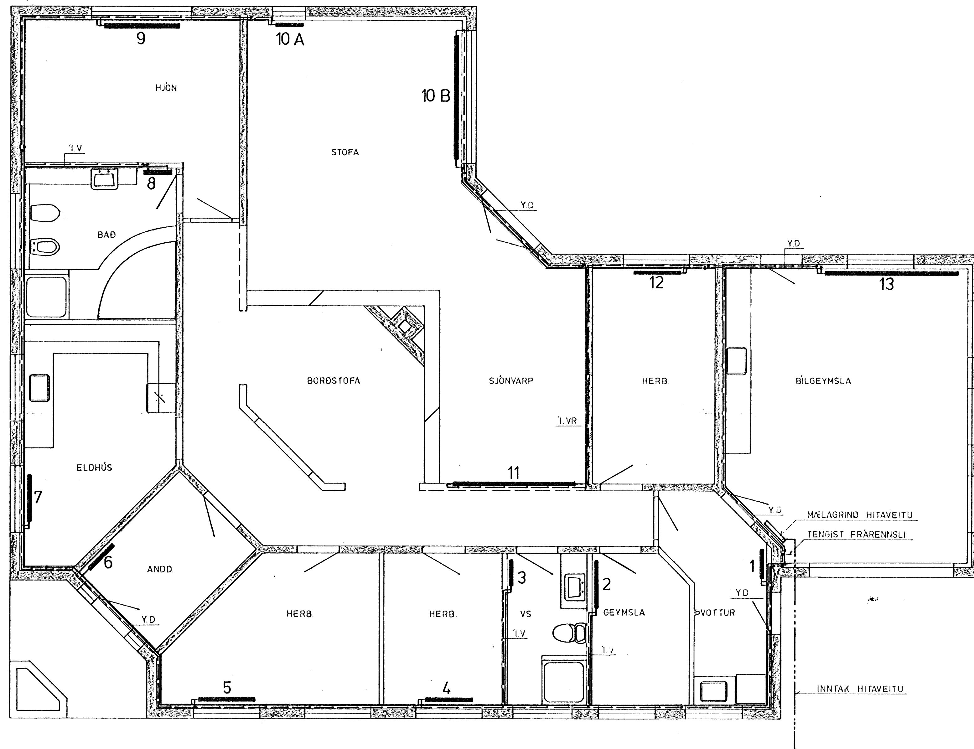
GRUNNMYND 1 : 50
