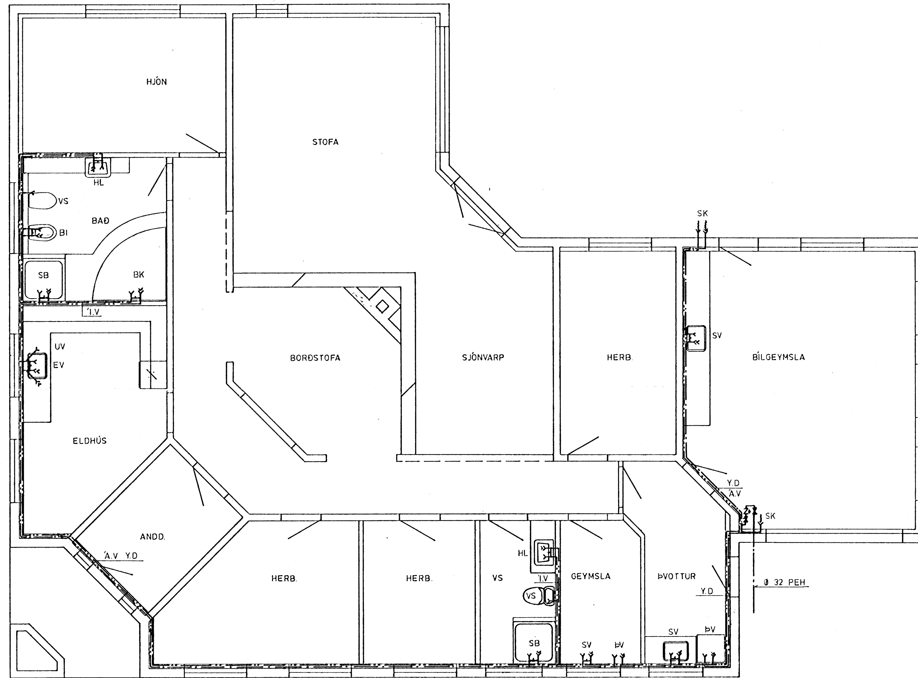
GRUNNMYND 1 : 50
