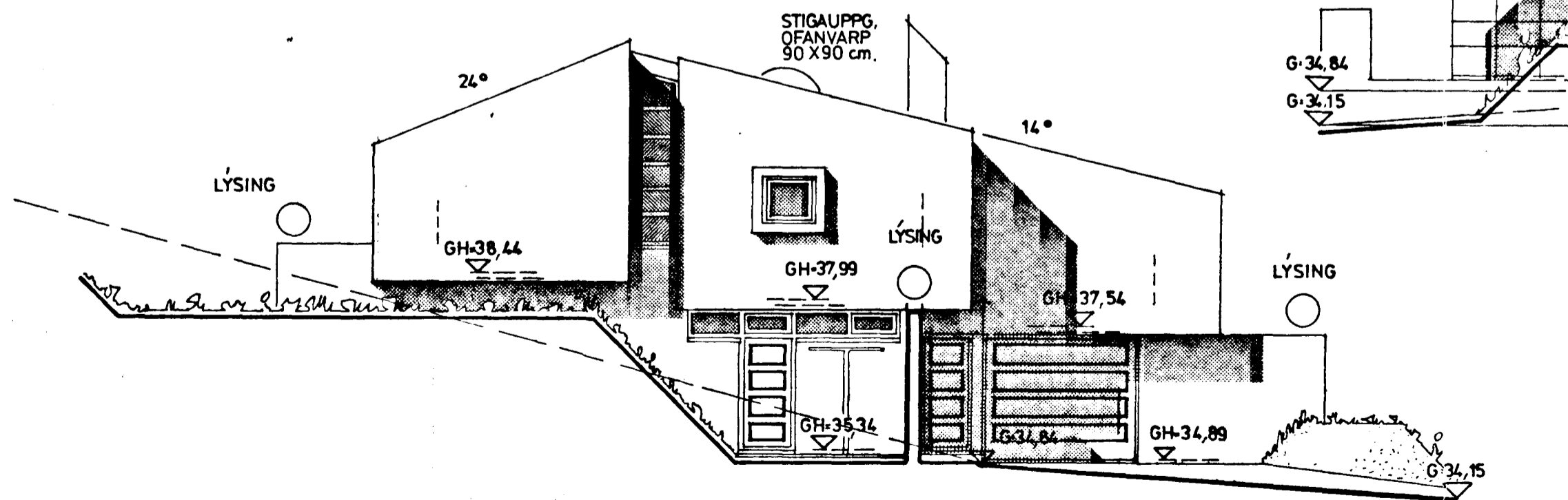
ÚTLIT, AUSTUR - GÖTUHLÍÐ
