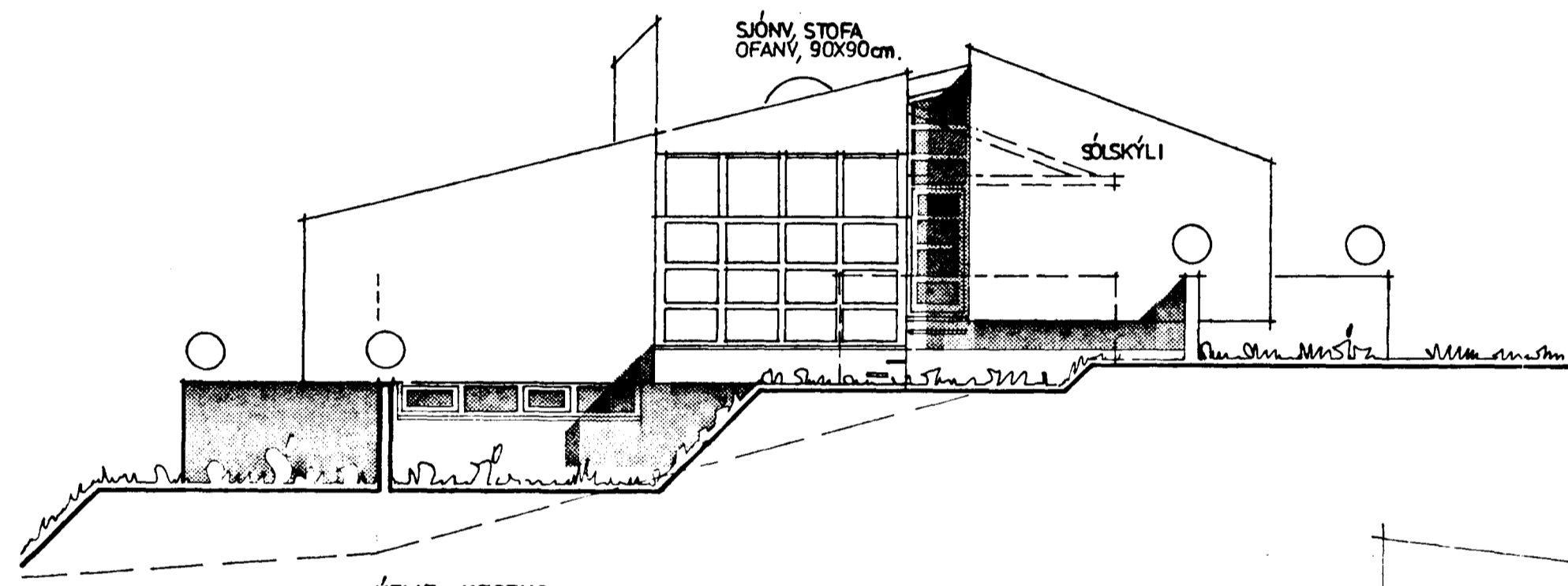
ÚTLIT, VESTUR
