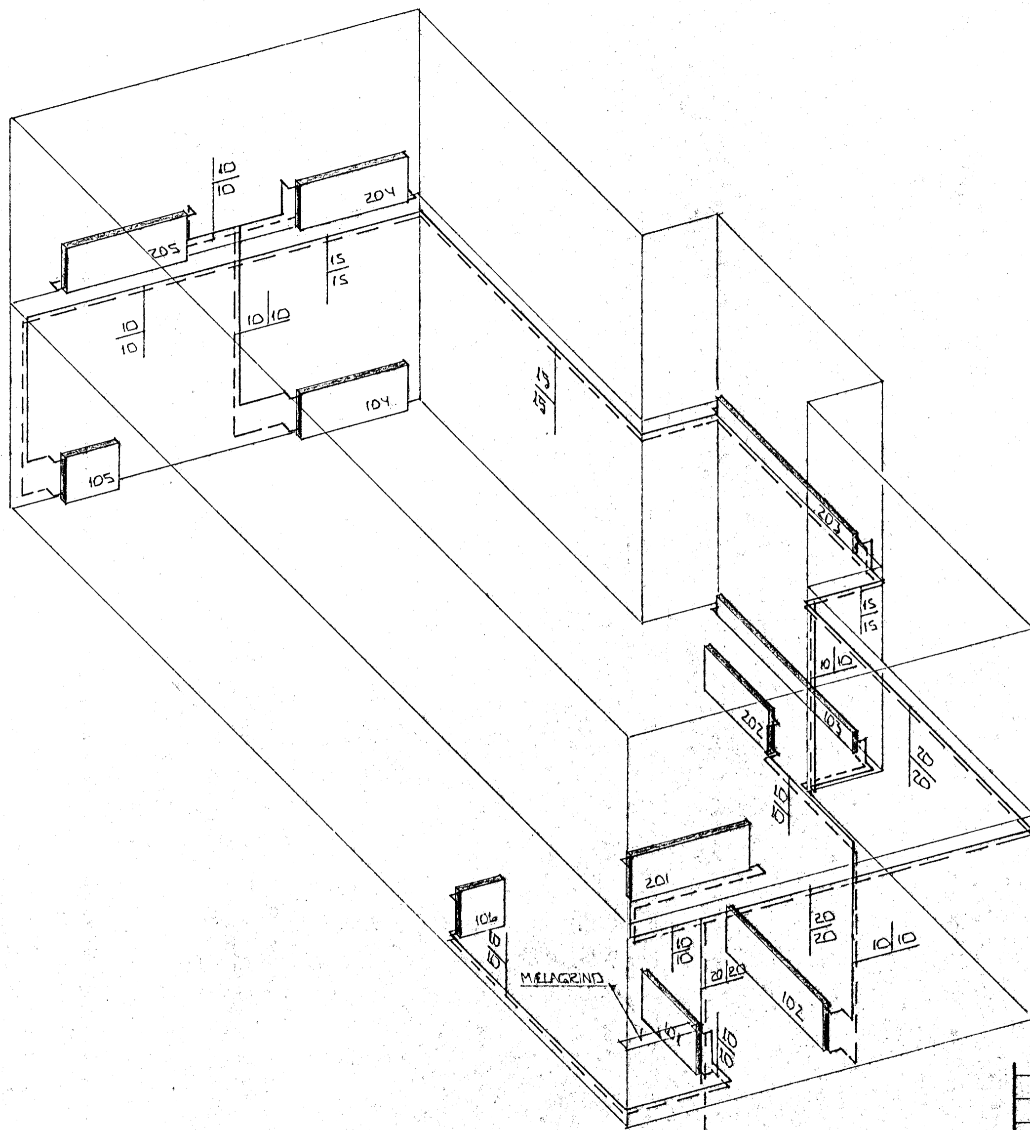
RÜMMYND HITALAGNA 1:50
